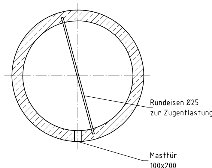
Schnitt D-D M. 1:33
