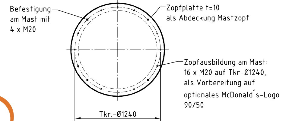
Draufsicht A M. 1:33 Zopfplatte als Abdeckung, für Mastzopf ohne McDonald's-Logo 90/50 Diese Version kommt vorerst zur Ausführung.
