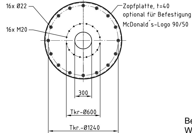
Schnitt A-A M. 1:33 Zopfplatte zur später möglichen Befestigung des McDonald's-Logos 90/50, nachrüstbar für Zopfausbildung 16xM20
