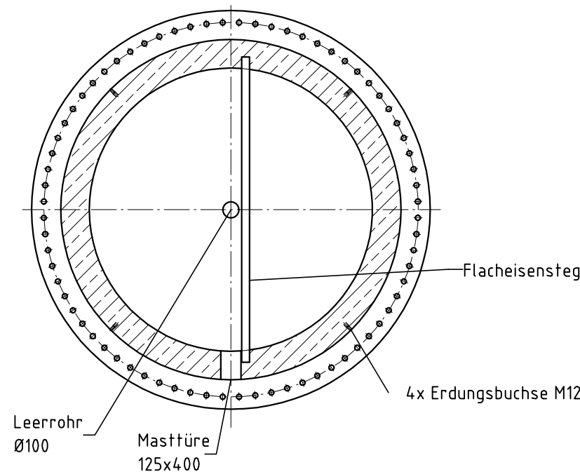
Schnitt D-D M. 1:33
