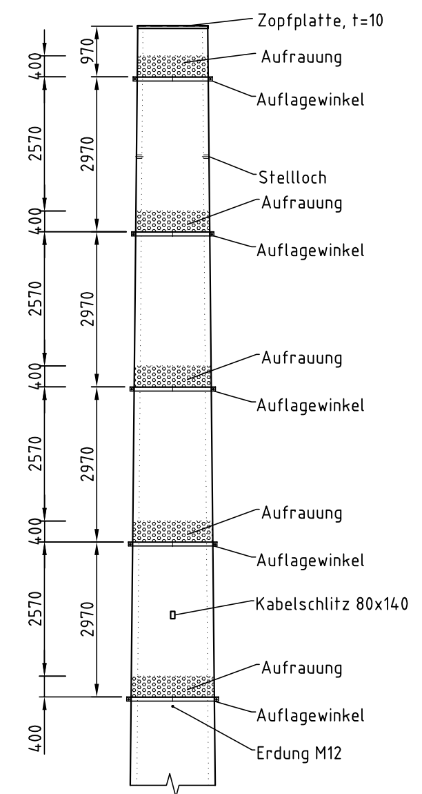
Anbindung Werbung dreieckig M. 1:100
