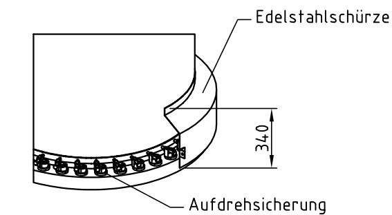
Edelstahlschürze
