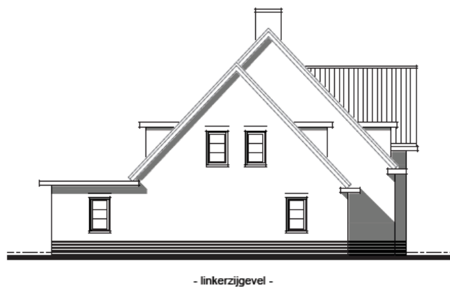
Figuur 4: Schetsontwerp.
