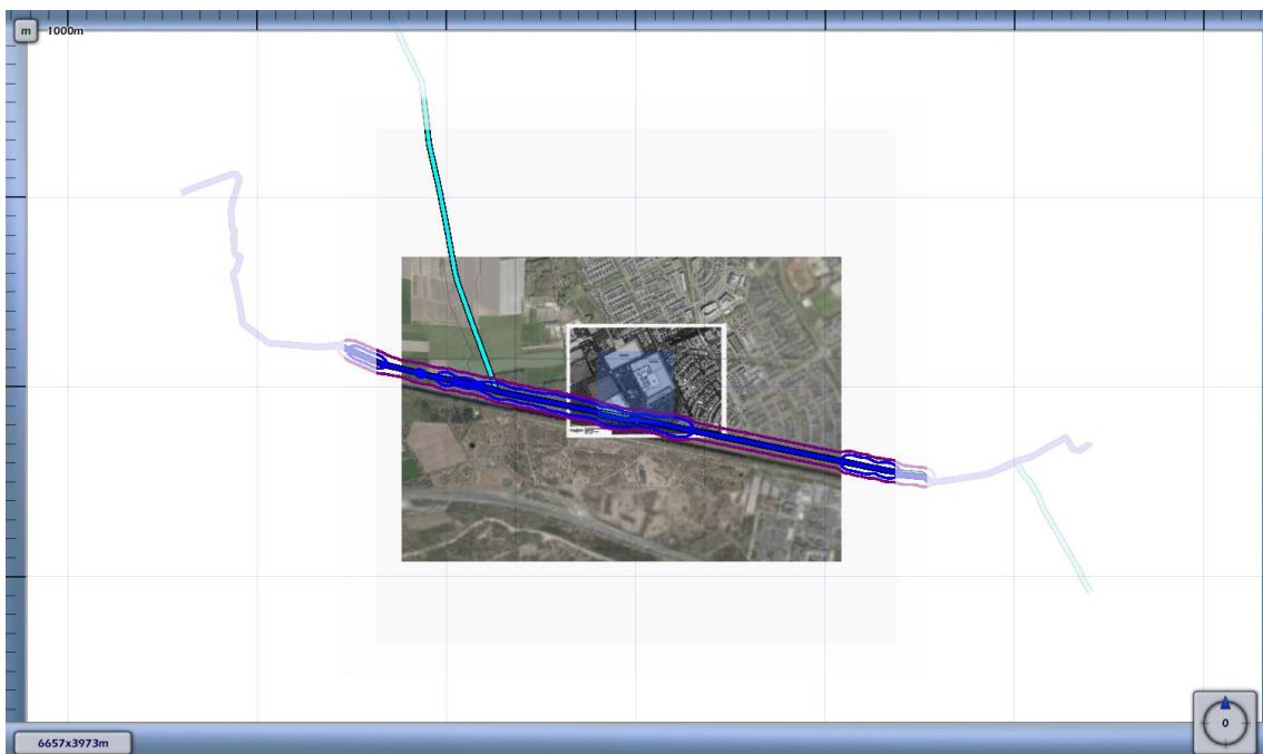
3.2 Figuur 3.2 Plaatsgebonden risico voor 8245_leiding-Z-510-28-deel-1 van N.V. Nederlandse Gasunie
