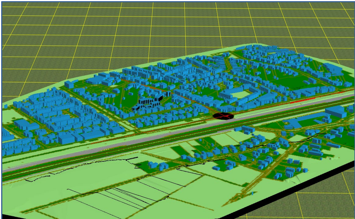
Afbeelding 4. Rekenmodel wegverkeerslawaaai, 3d-weergave (totaal)
