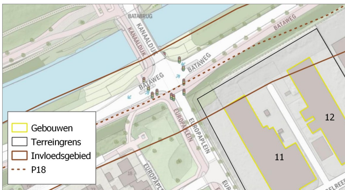
Figuur 3. Invloedsgebied kerosineleiding
