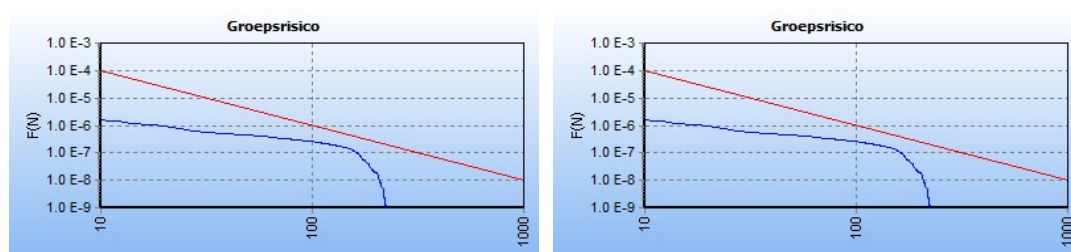
Figuur 6. Groepsrisico A-525-02, huidig (links) en toekomstig (rechts)
