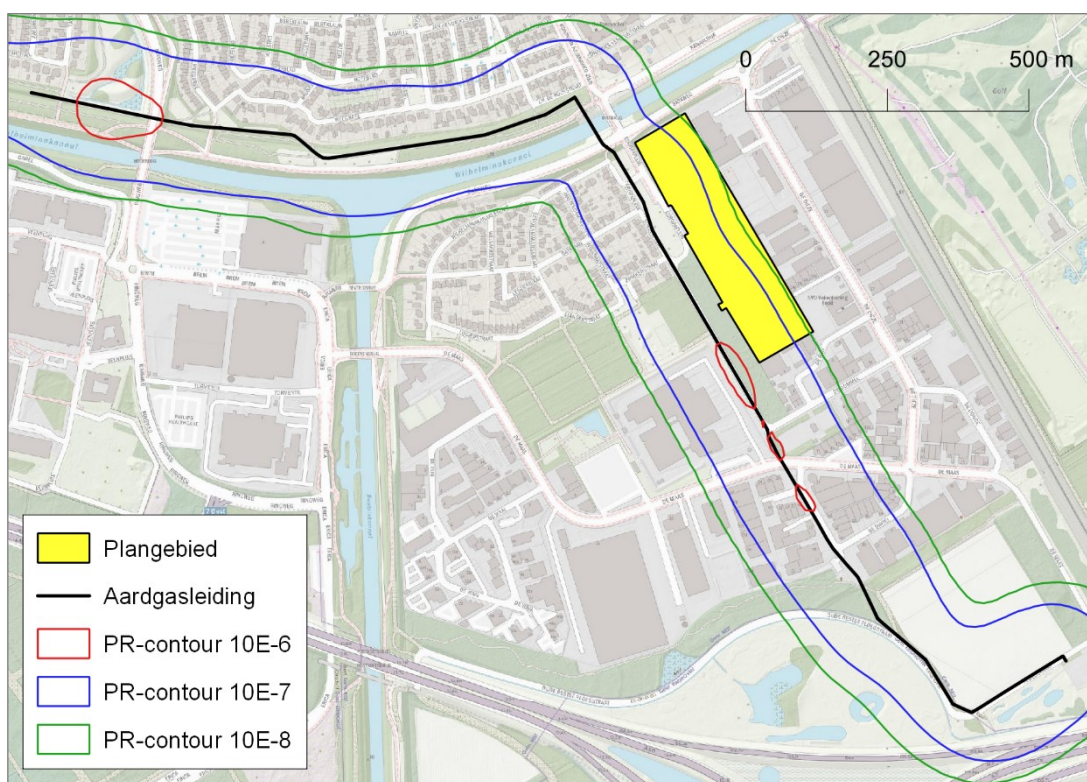
Figuur 5. Plaatsgebonden risicocontouren aardgasbuisleiding A-525-02
