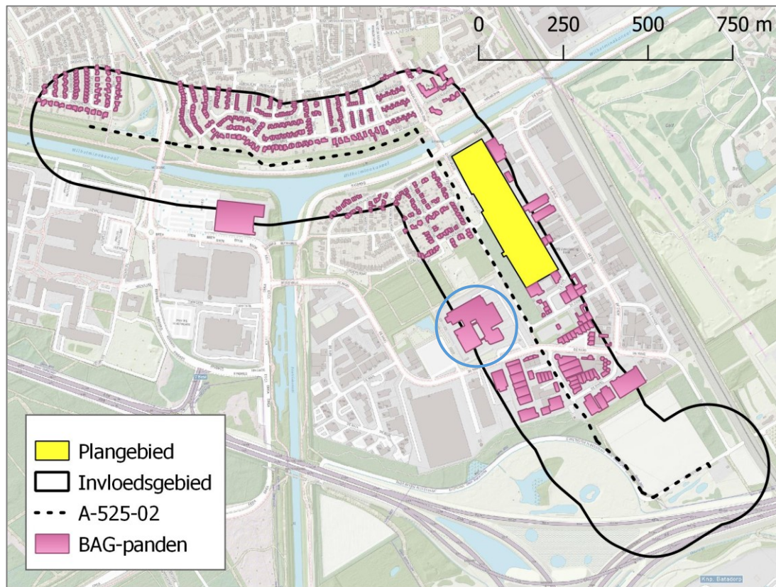
Figuur 8. Bebouwing binnen invloedsgebied aardgasleiding ○ Van grote invloed op het groepsrisico
