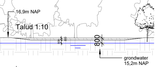
2 Doorsnede 1 1 : 300
