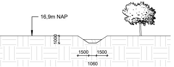
3 Doorsnede 2 1 : 300
