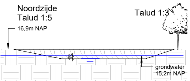
4 Doorsnede 3 1 : 300
