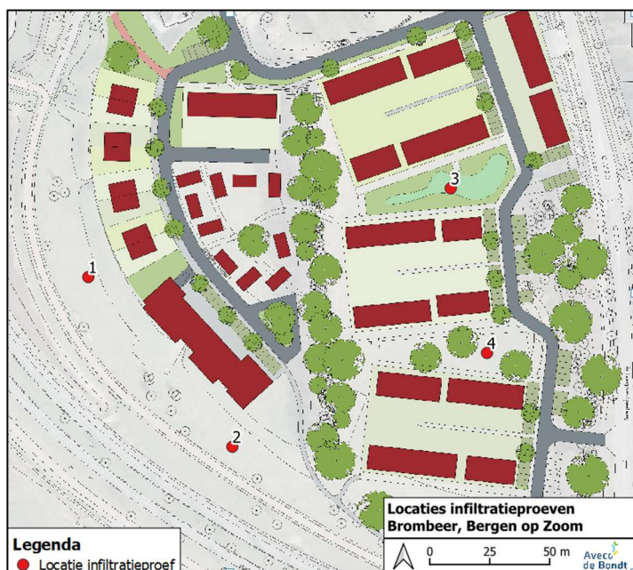
Figuur 4 – Overzichtstekening infiltratieproeven en bodemonsters
