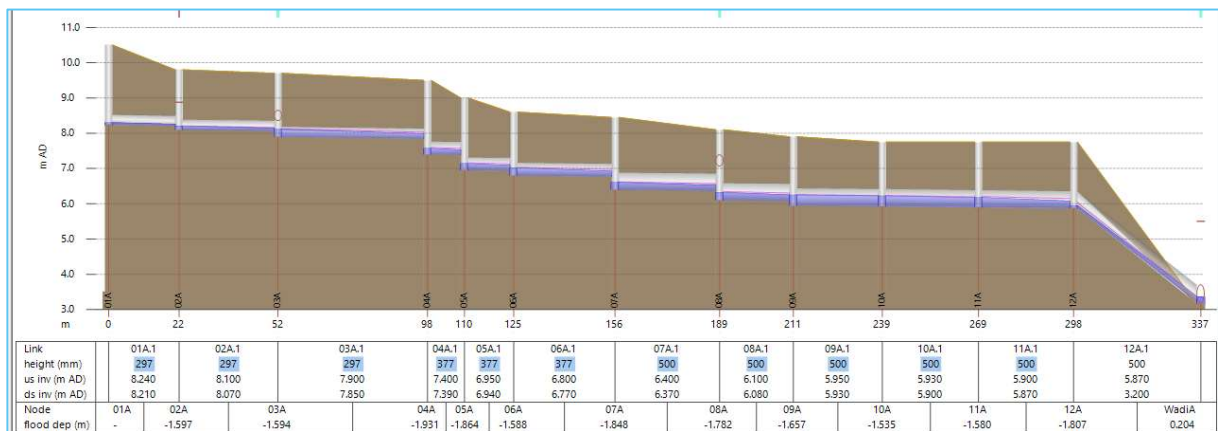
Figuur 7 – Dwarsdoorsnede pieksituatie Bui08
