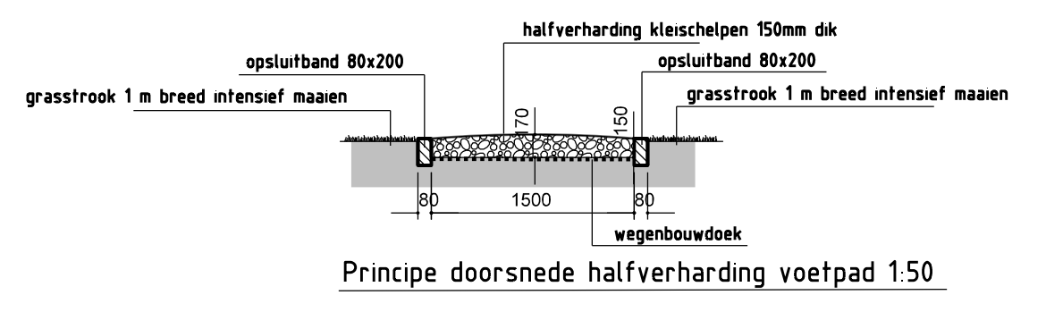
Doorsnede D 150
