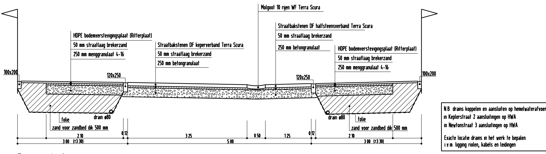
Doorsnede A 150
