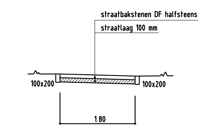
Doorsnede C 150
