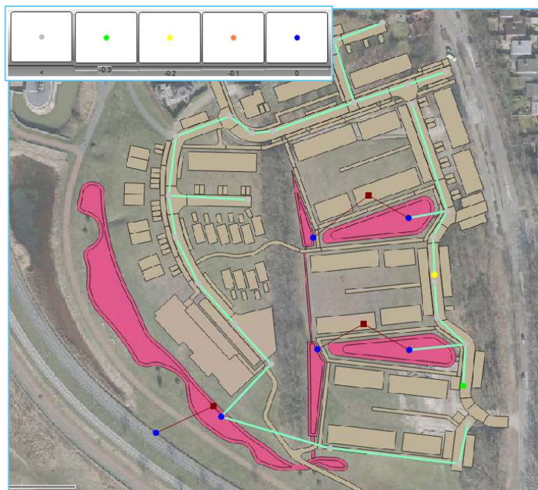
Figuur 8 – Bovenaanzicht hydraulische toetsing plangebied Bui10
