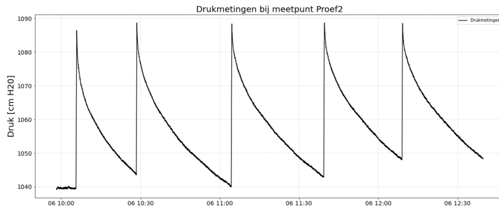
Figuur B Meetreeks proeven meetpunt 2
