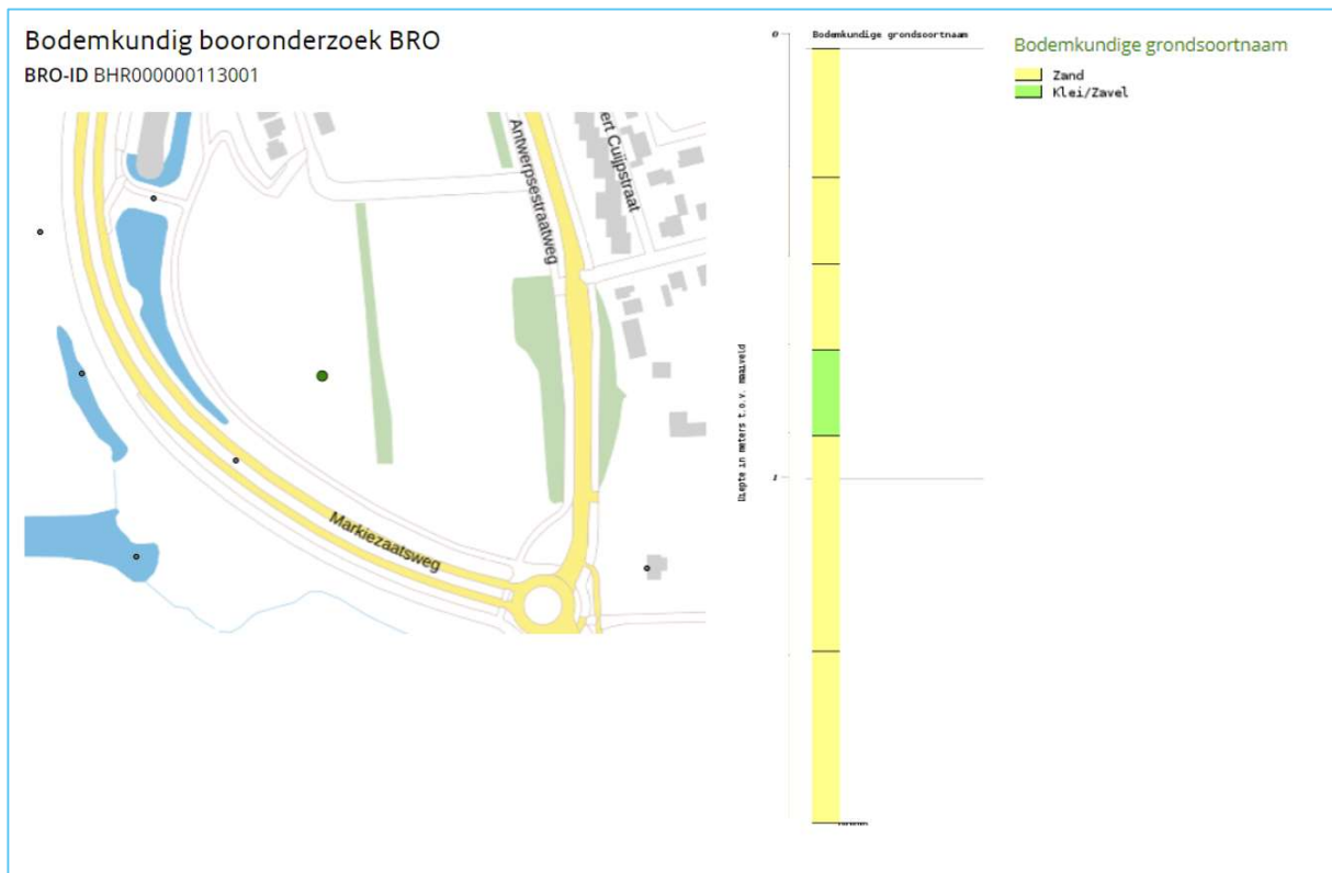
Figuur 2 – Bodemopbouw boring BHR0000000113001
