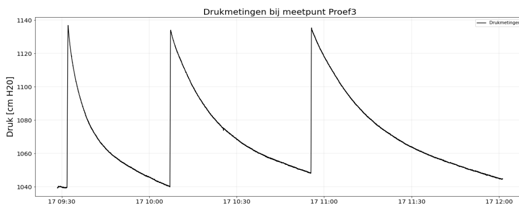
Figuur C Meetreeks proeven meetpunt 3
