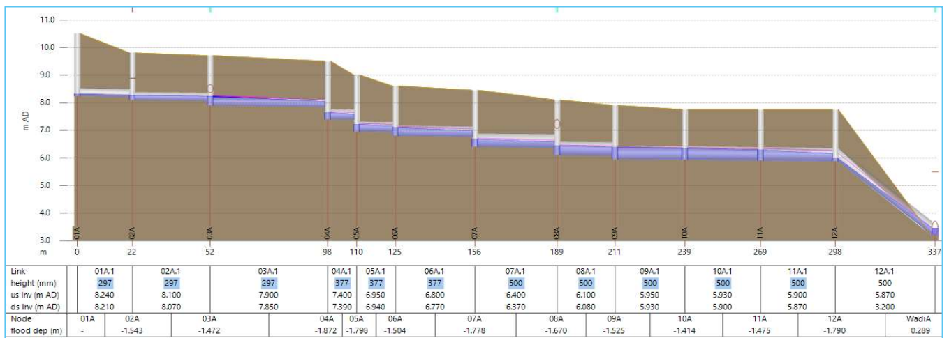
Figuur 9 – Dwarsdoorsnede pieksituatie Bui10
