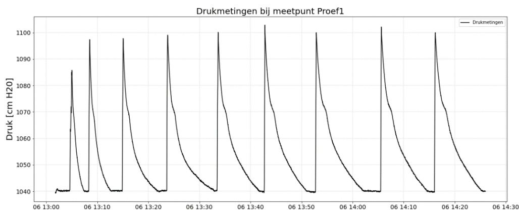
Figuur A Meetreeks proeven meetpunt 1
