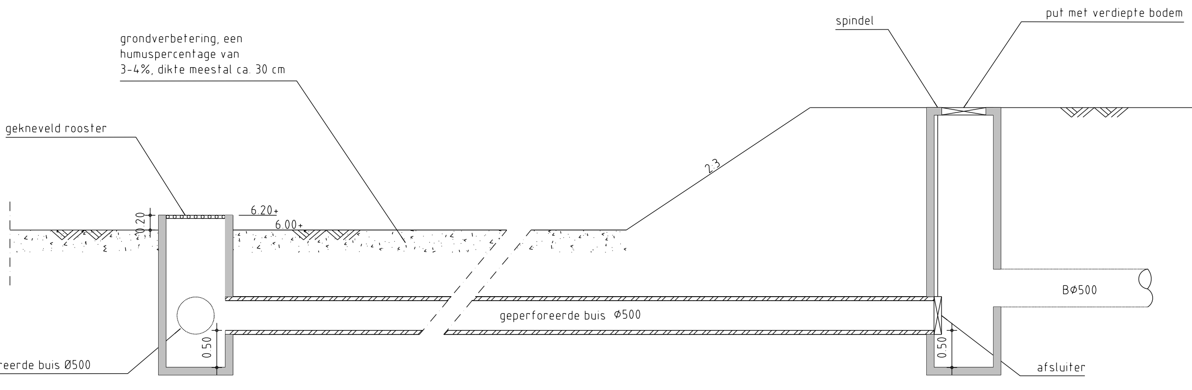
Principeddoorsnede Infiltratievoorziening 150
