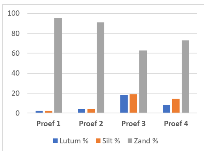
Figuur 2. Bodemopbouw volgens zeefkrommen.
