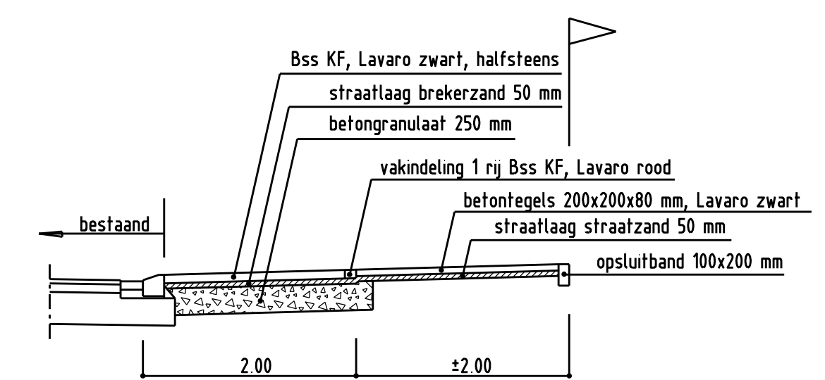
Doorsnede B 150
