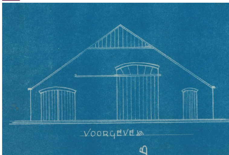
Ontwerp voorgevel 1941. Bron: Regionaal Archief Tilburg.
