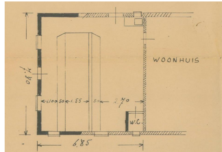
Ontwerp voor een aanbouw aan het woonhuis plattegrond, 1953. Bron: Regionaal Archief Tilburg.
