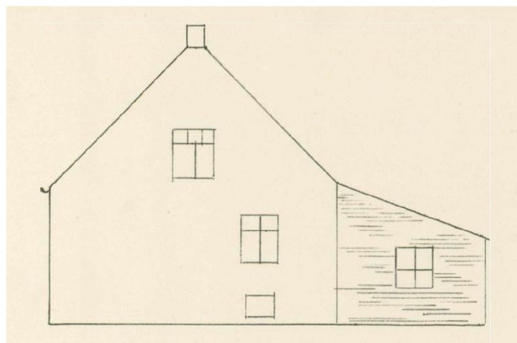
Ontwerp voor een aanbouw rechterzijgevel, 1964. Bron: Regionaal Archief Tilburg.
