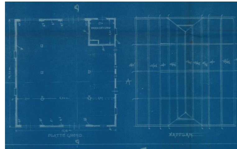
Ontwerp plattegrond en kapplan 1941. Bron: Regionaal Archief Tilburg.
