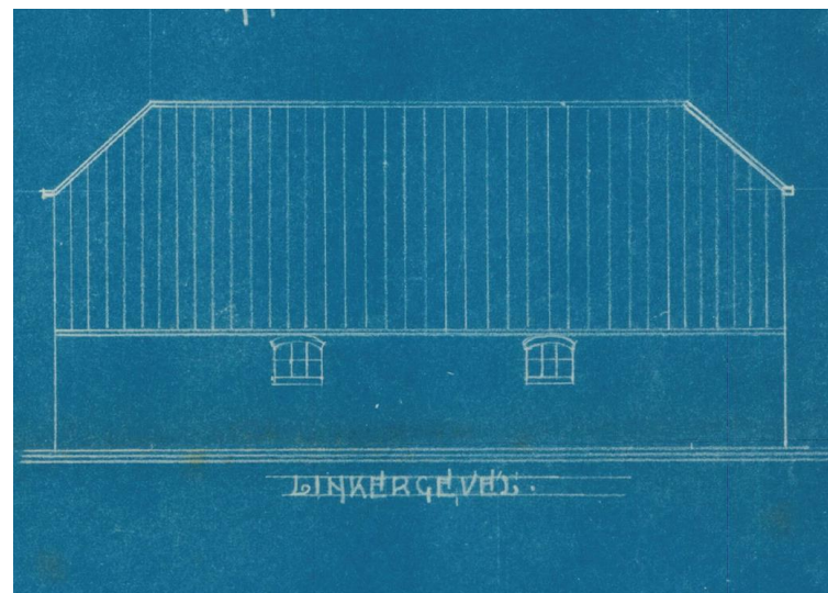
Ontwerp linkerzijgevel 1941. Bron: Regionaal Archief Tilburg.
