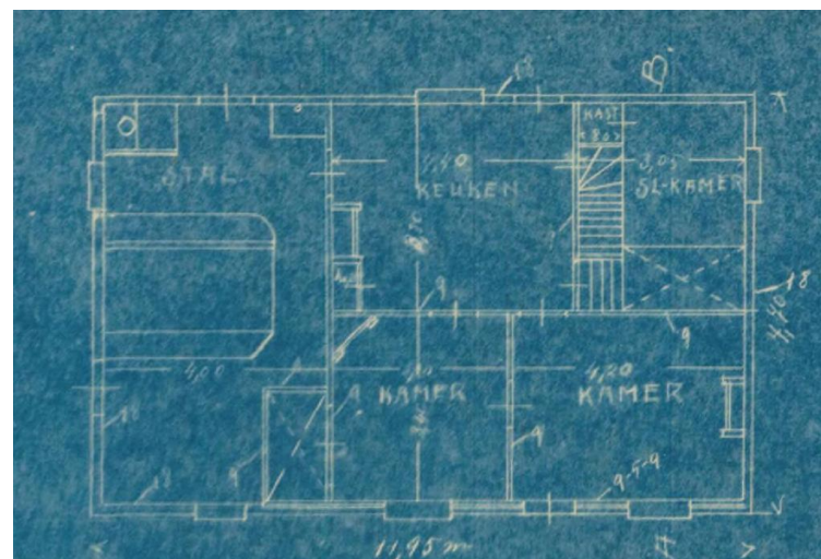
Ontwerp voor een nieuw te bouwen woonhuis plattegrond, 1931. Bron: Regionaal Archief Tilburg.
