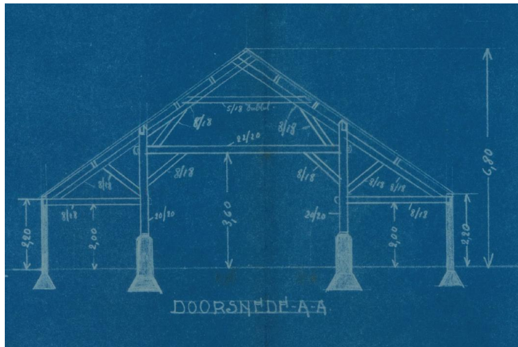
Ontwerp doorsnede A-A 1941. Bron: Regionaal Archief Tilburg.
