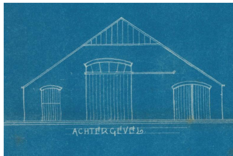
Ontwerp achtergevel 1941. Bron: Regionaal Archief Tilburg.
