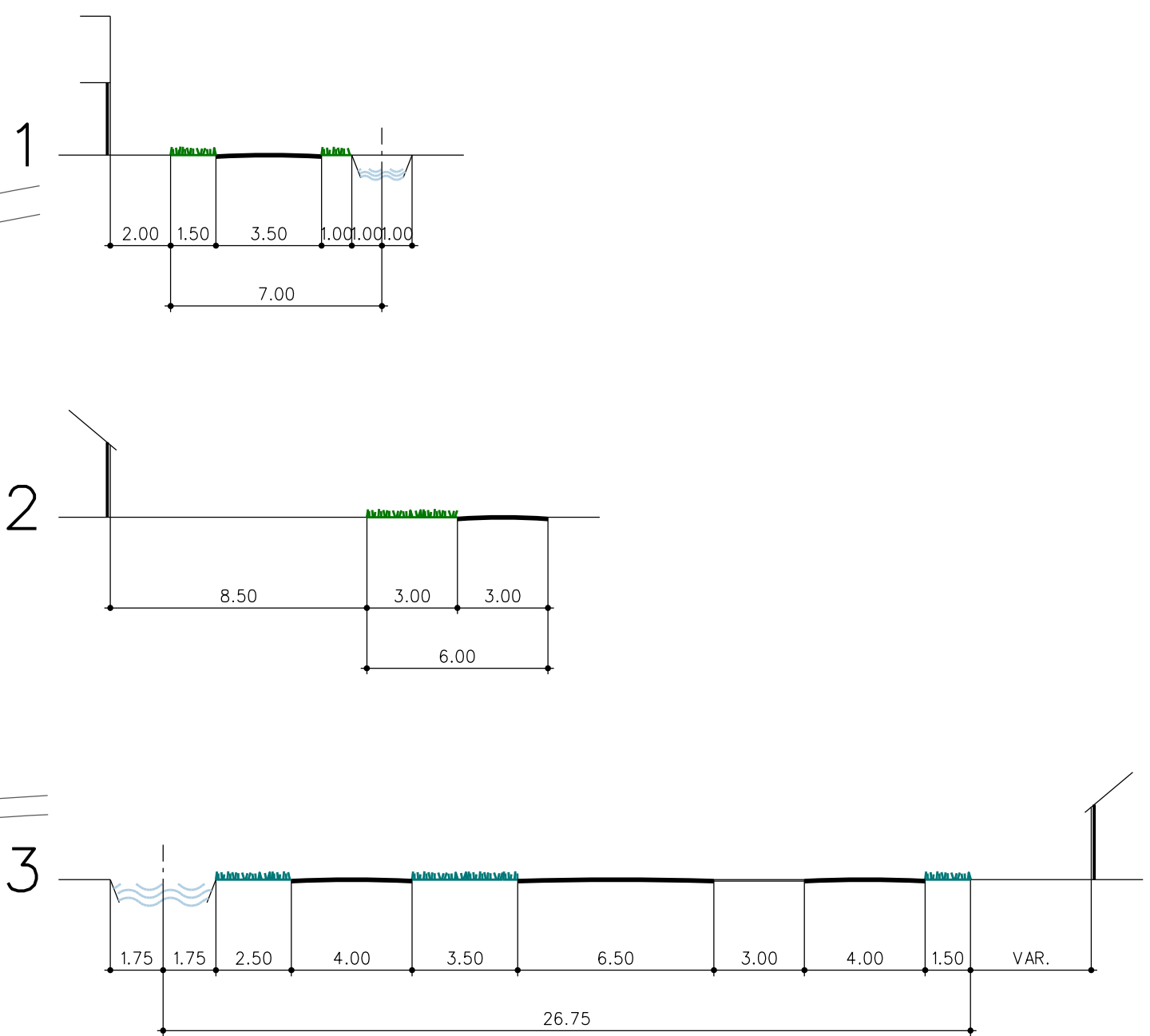
DWARSPROFIELEN SCHAAL 1:200
