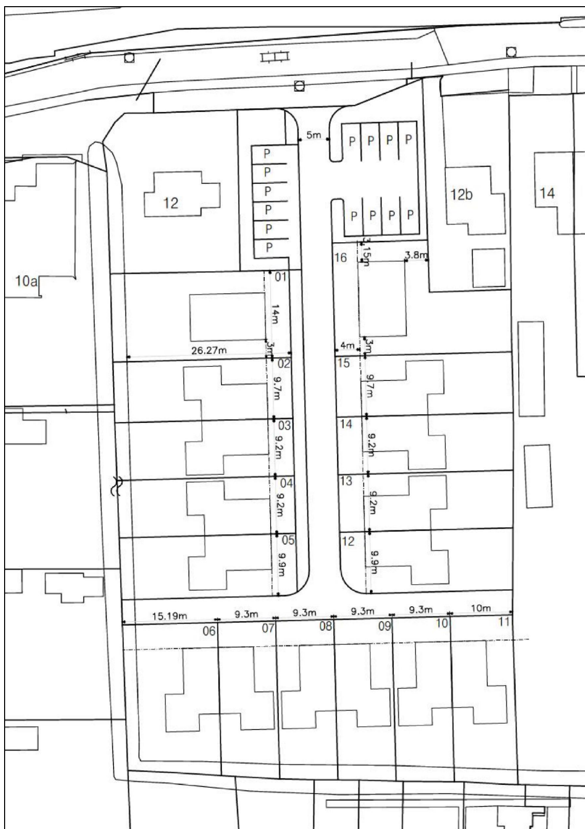
Figuur 3. Impressie van de plansituatie Rijksstraatweg 12 te Hurdegaryp.
