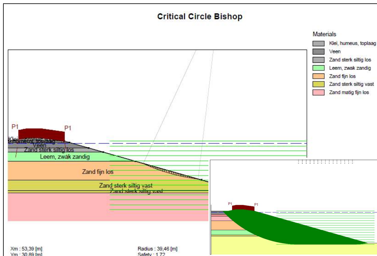
Figuur 3-1: Resultaat veiligheid tegen afschuiven.
