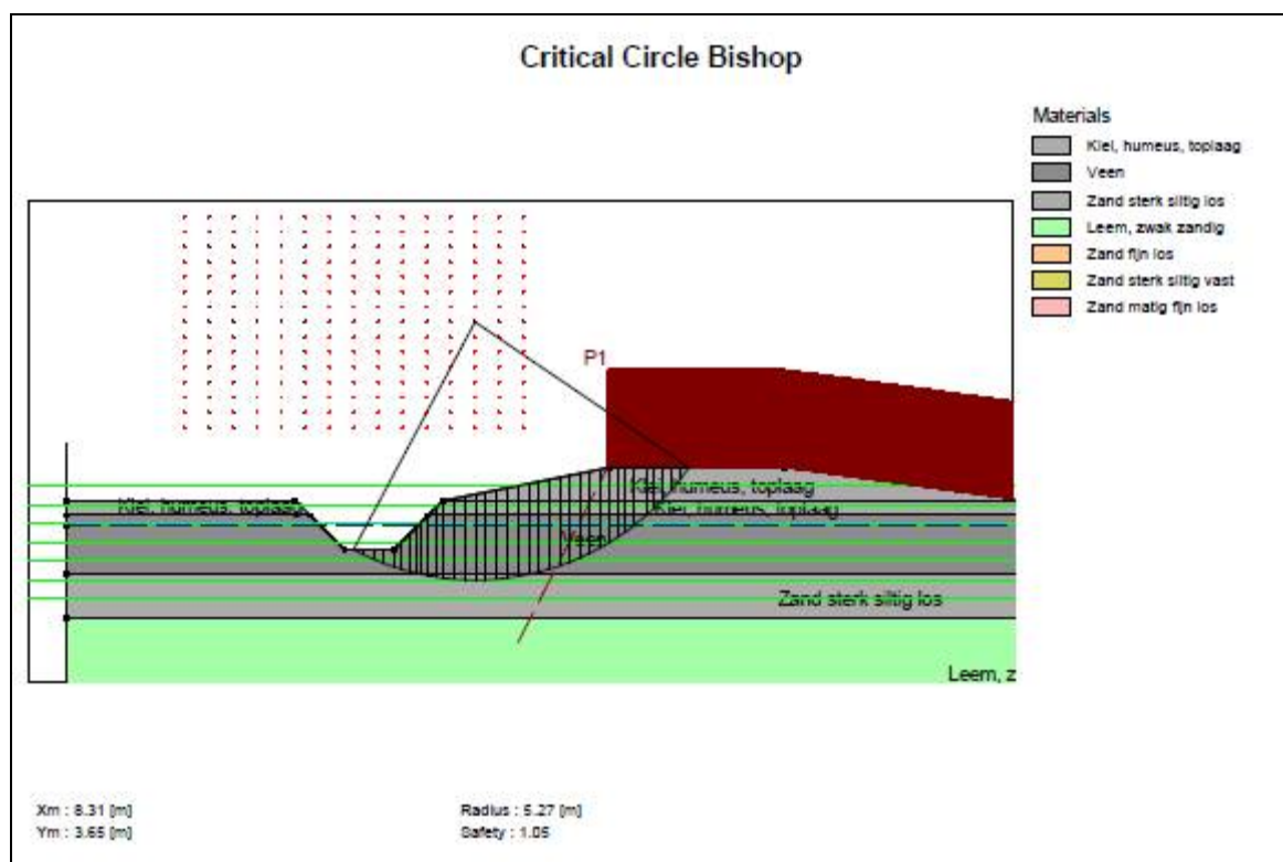
Figuur 4.1 : Stabiliteitsanalyse sloot
