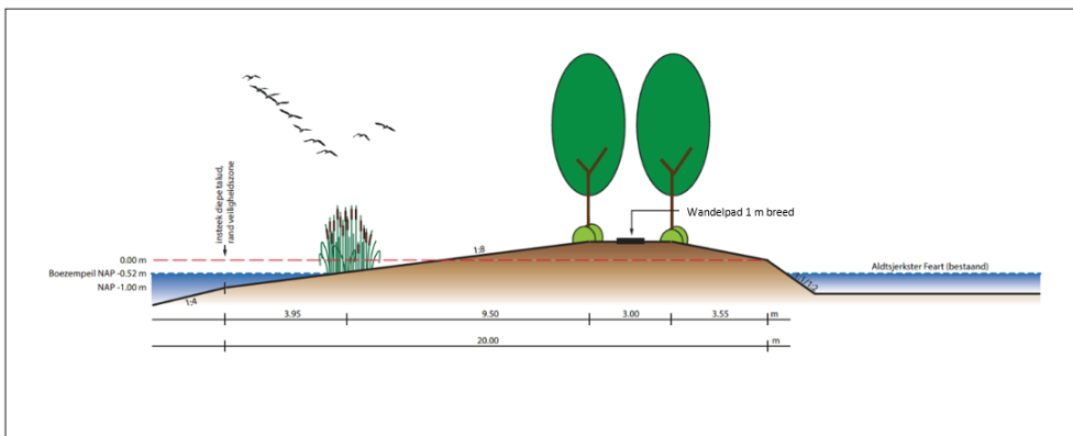
Oeverprofiel zuidzijde zandwinning (aangepaste tekening Sweco uit 2017)
