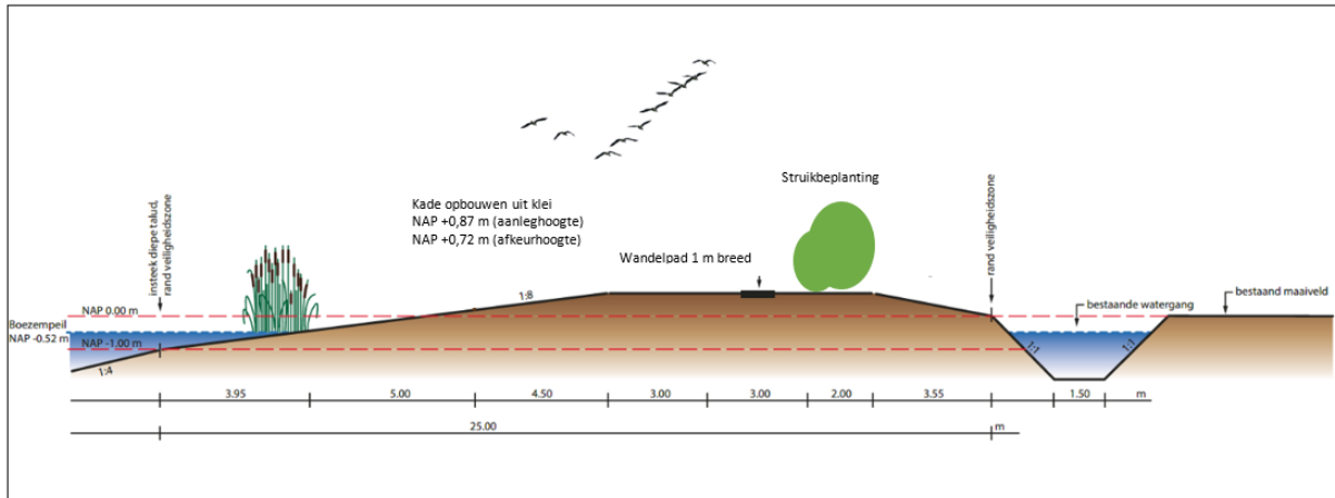
Oeverprofiel noordzijde zandwinning (aangepaste tekening Sweco uit 2017)
