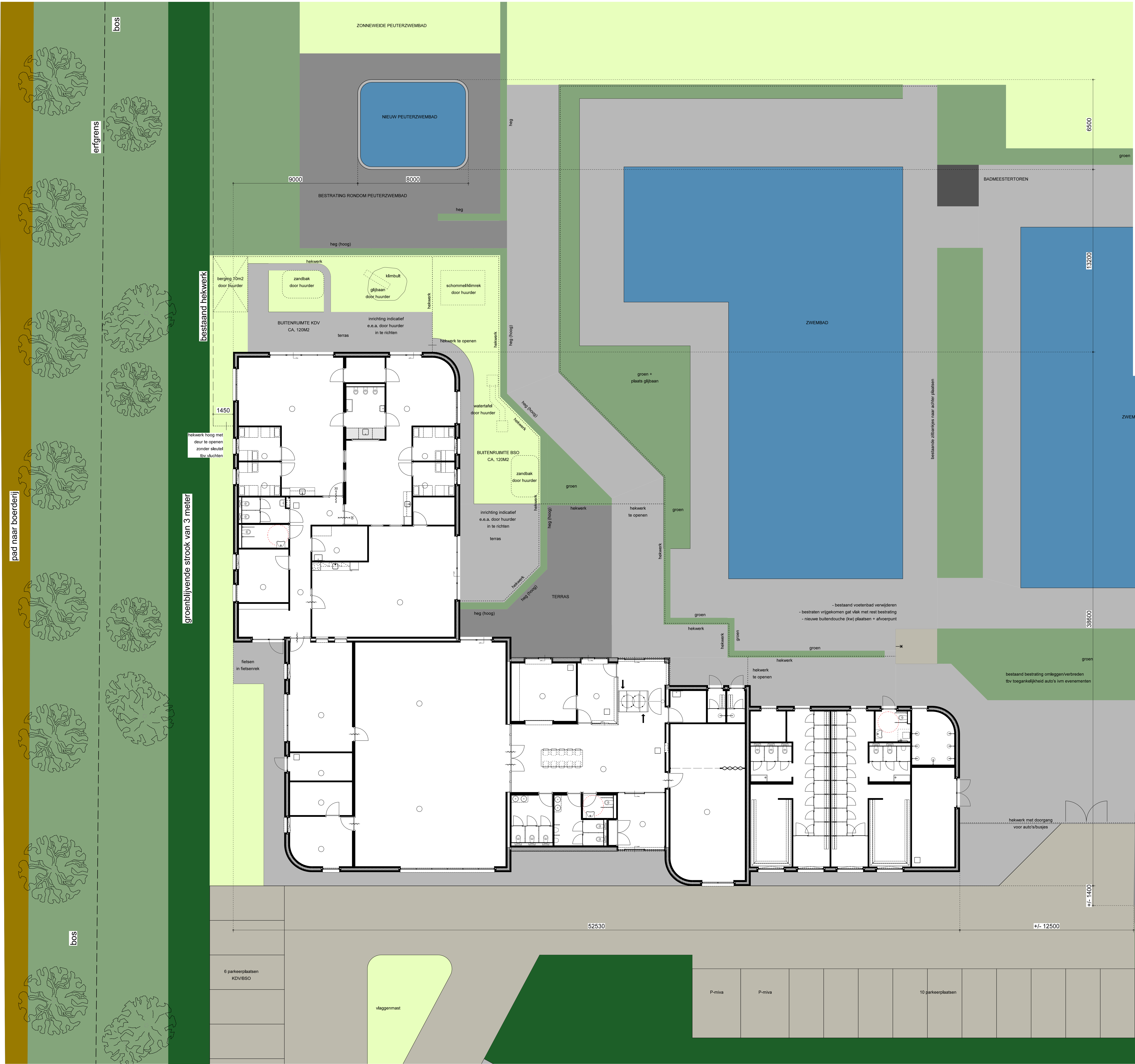
TERREINPLAN (DEELS) 1:100
