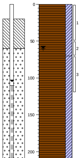
Boring: 101 Datum: 18-10-2022 Boormeester: Gerben van Dasselaar
