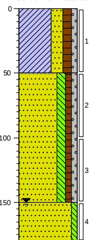
Boring: 105 Datum: 18-10-2022 Boormeester: Gerben van Dasselaar
