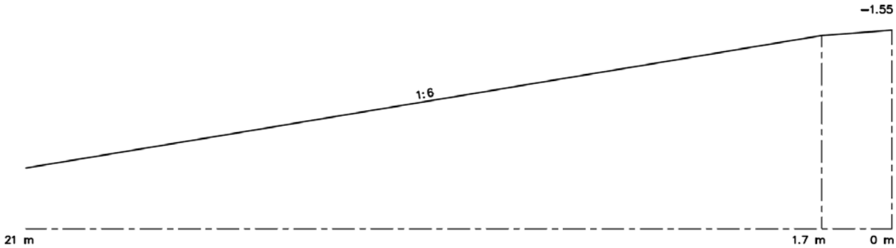
DWARSPROFIEL
