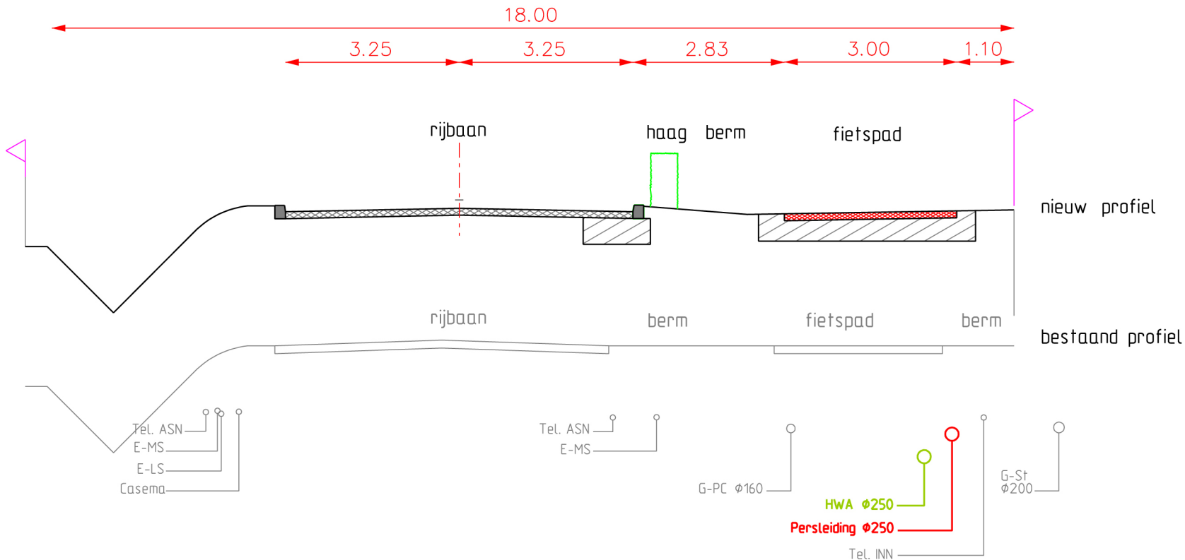
Dwarsprofiel 2
