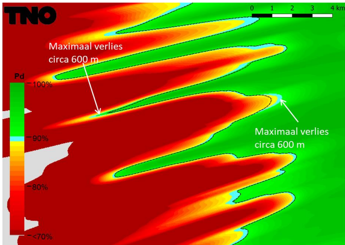
Figuur 12 Het gebied waar door de schaduwwerking op de radar bij Wemeldingen een verlies aan bereik optreedt uit figuur 11 groter weergegeven, dus nadat het bouwplan is gerealiseerd. De zwart gestippelde lijn geeft het oorspronkelijke bereik aan zonder het bouwplan.
