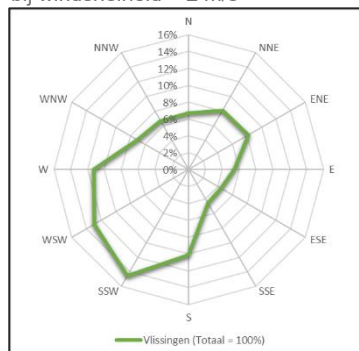
Figuur 3.2 Distributie windrichtingen bij windsnelheid > 2 m/s
