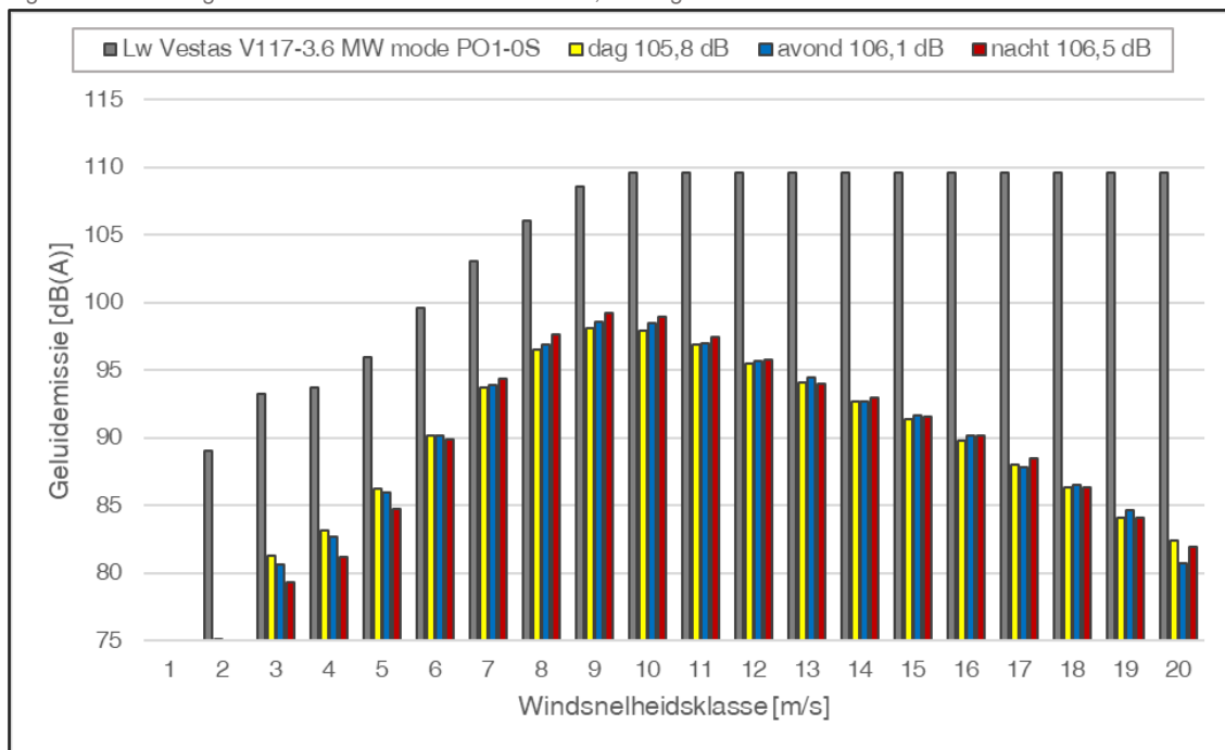
Figuur 2.2 Verdeling bronsterkten worst-case windturbine, ashoogte 117 m
