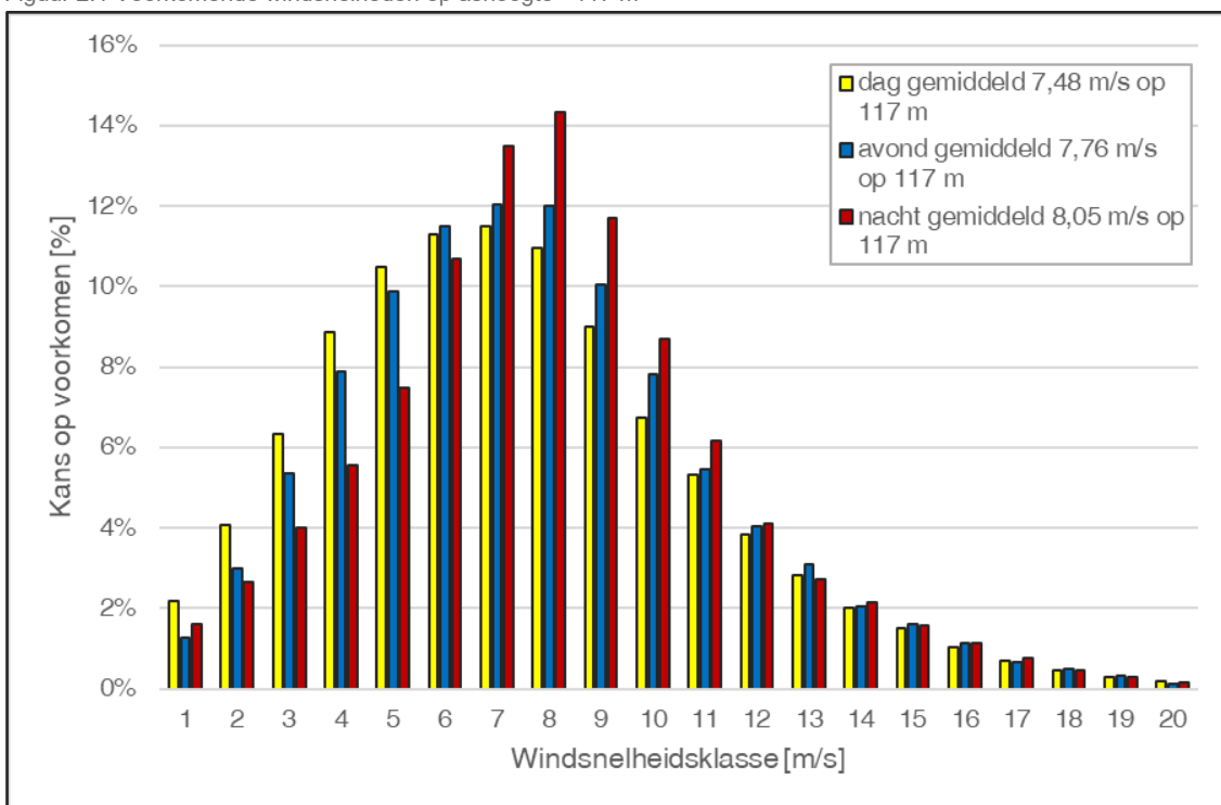
Figuur 2.1 Voorkomende windsnelheden op ashoogte +117 m
