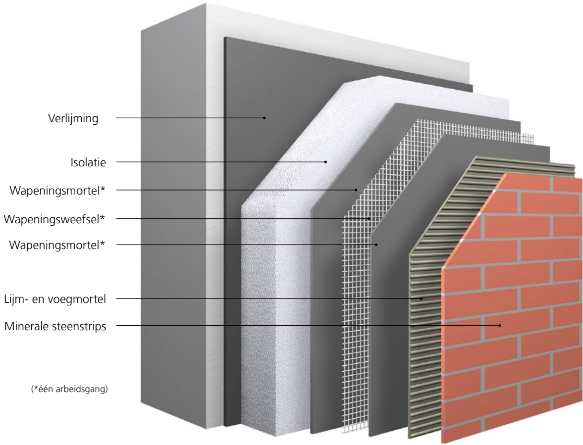
Systeemopbouw StoTherm Classic met minerale Sto-Steenstrips
