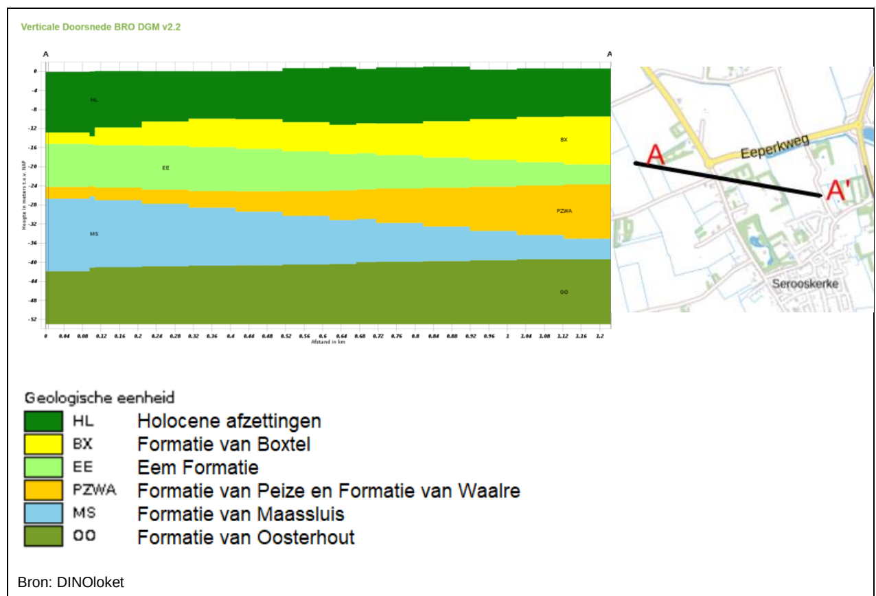
Figuur 2: verticale doorsnede Oostkapelseweg 32 te Serooskerke (BRO DGM v 2.2)
