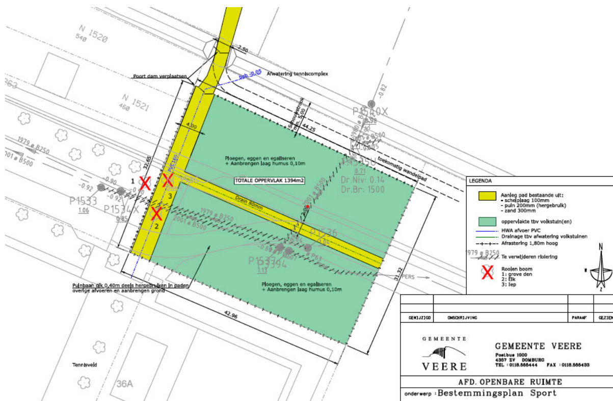
Figuur 2 Inrichtingsplan voor de volkstuinten
