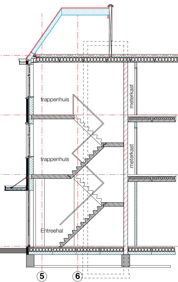
Trappenhuis
