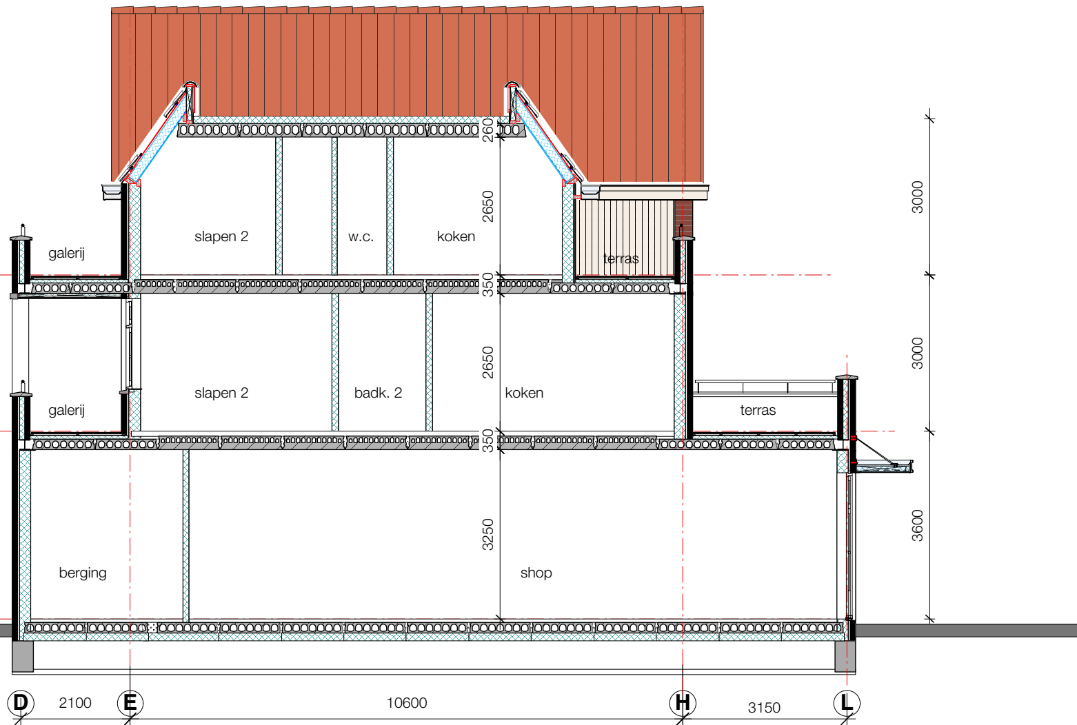
Doorsnede E-E
