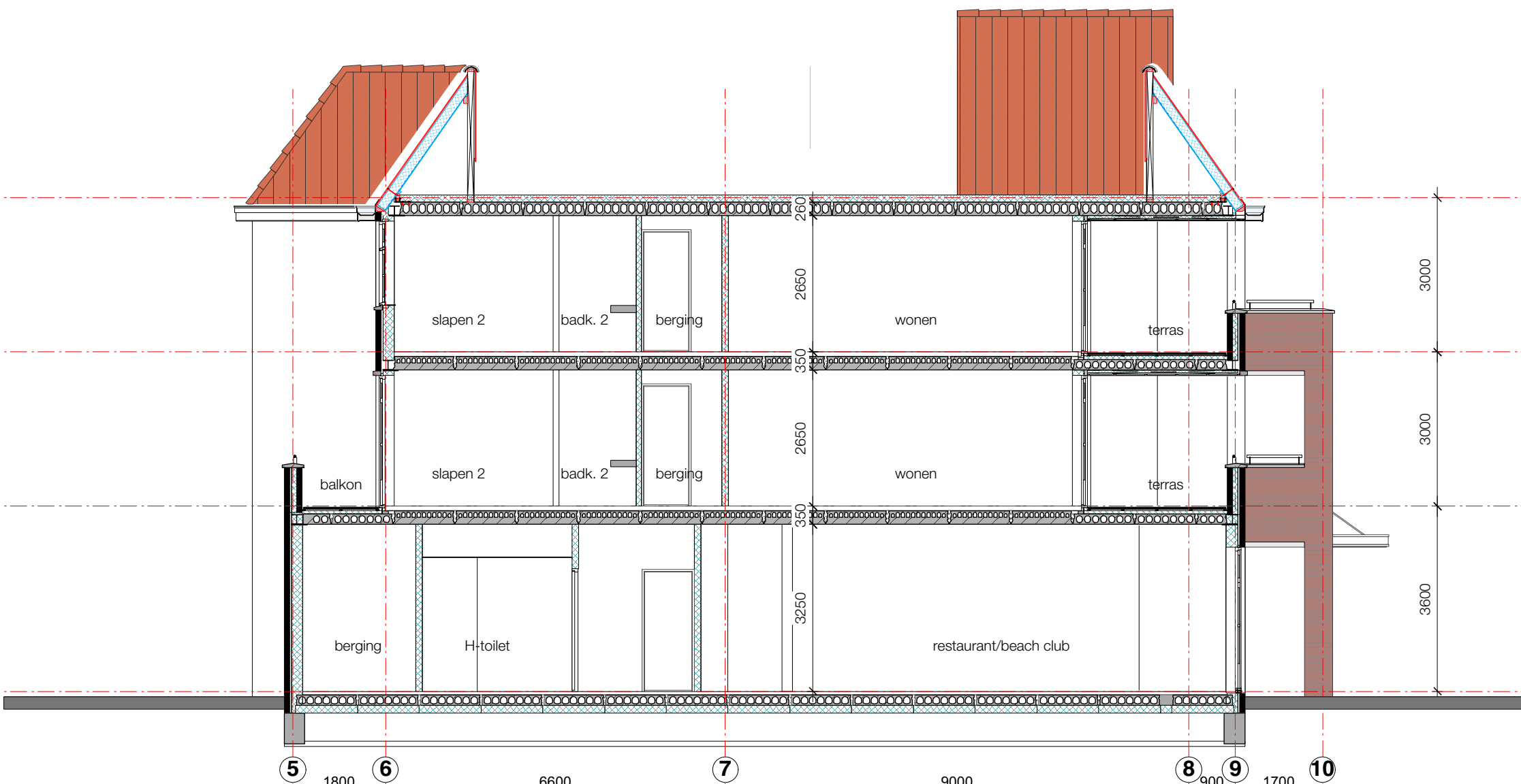
Doorsnede D-D
