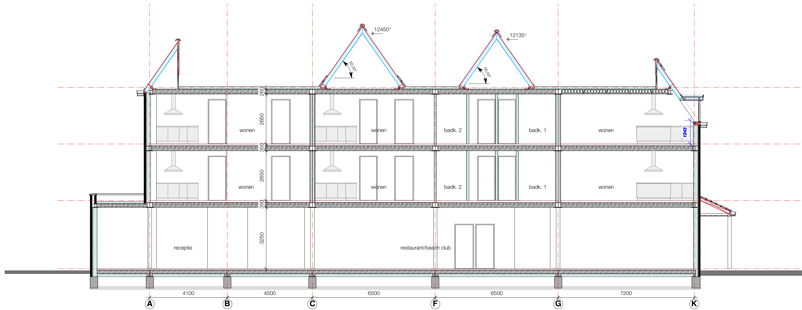
Doorsnede A-A
