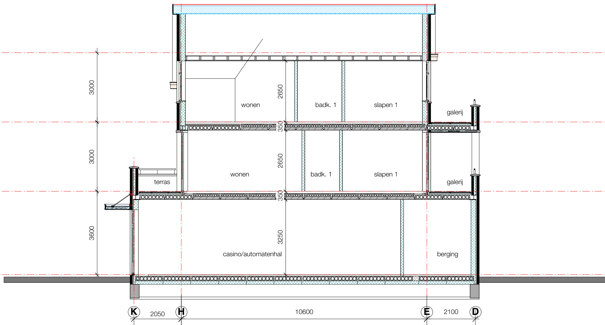
Doorsnede B-B
