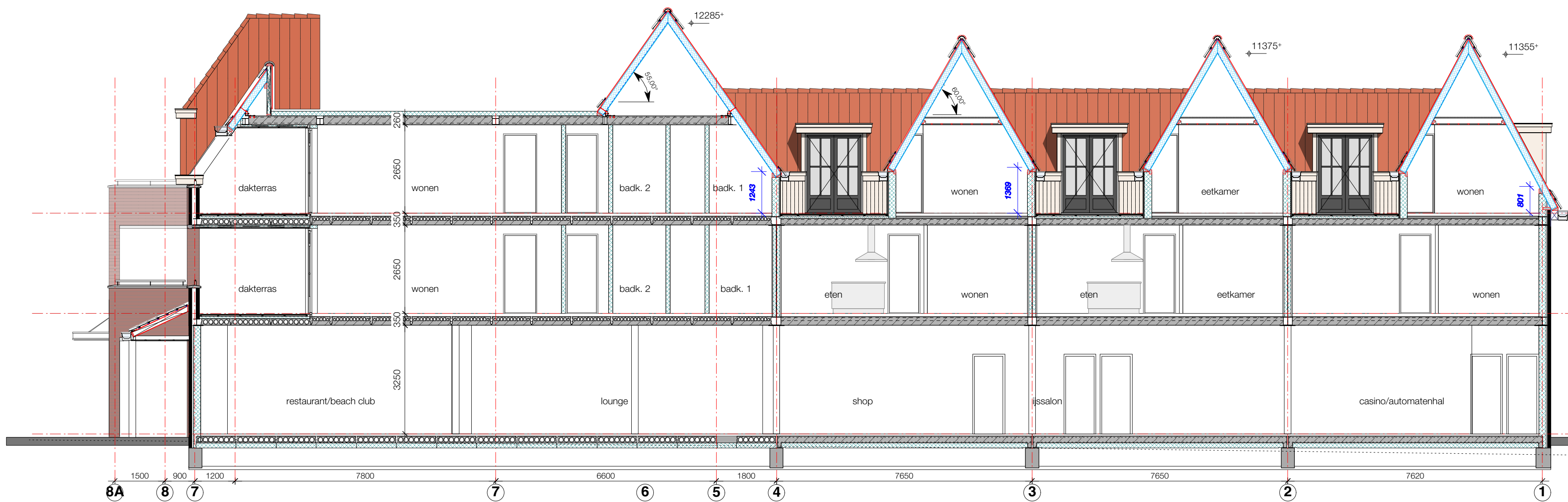
Doorsnede C-C
