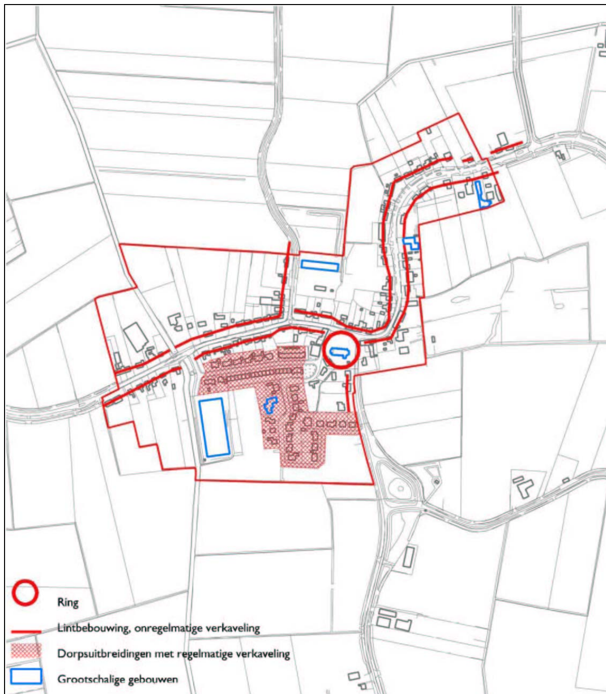
Figuur 3: Ruimtelijke hoofdstructuur
