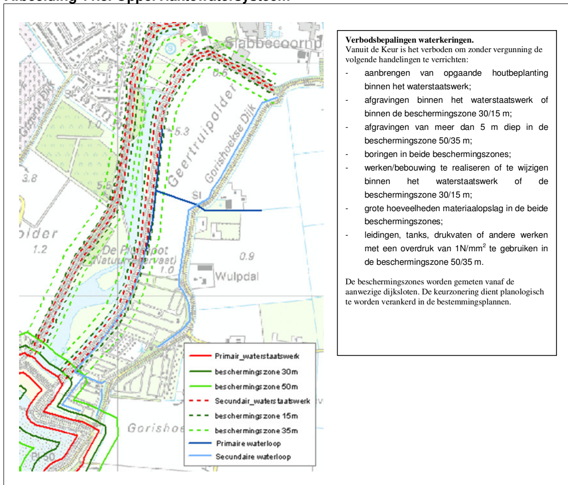
Afbeelding 11.3. Oppervlaktewatersysteem
