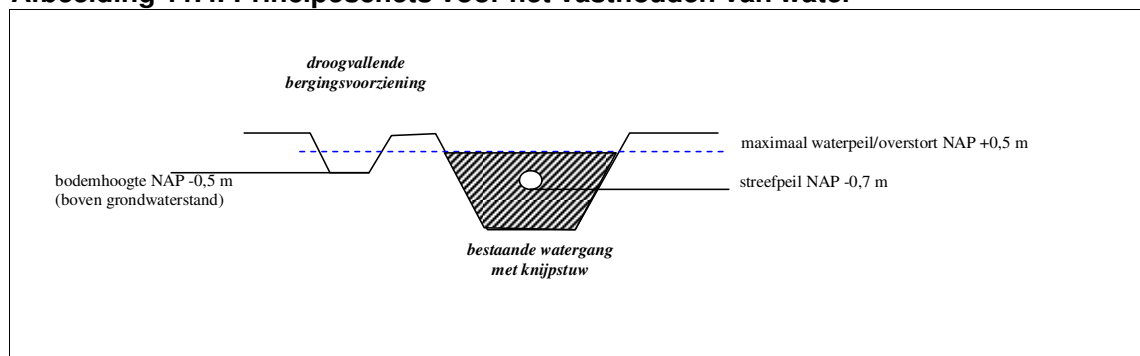
Afbeelding 11.4. Principeschets voor het vasthouden van water
