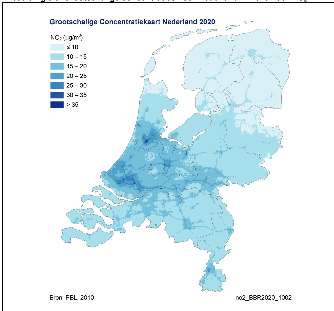
Afbeelding 8.5. Grootschalige concentraties voor Nederland in 2020 voor NO 2
