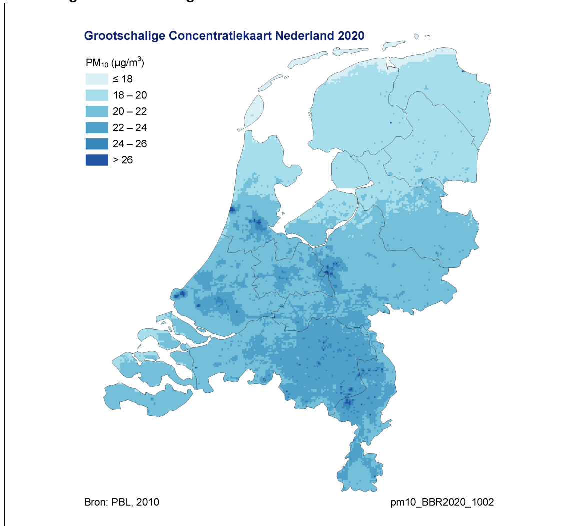
Afbeelding 8.4. Grootschalige concentraties voor Nederland in 2020 voor PM10
