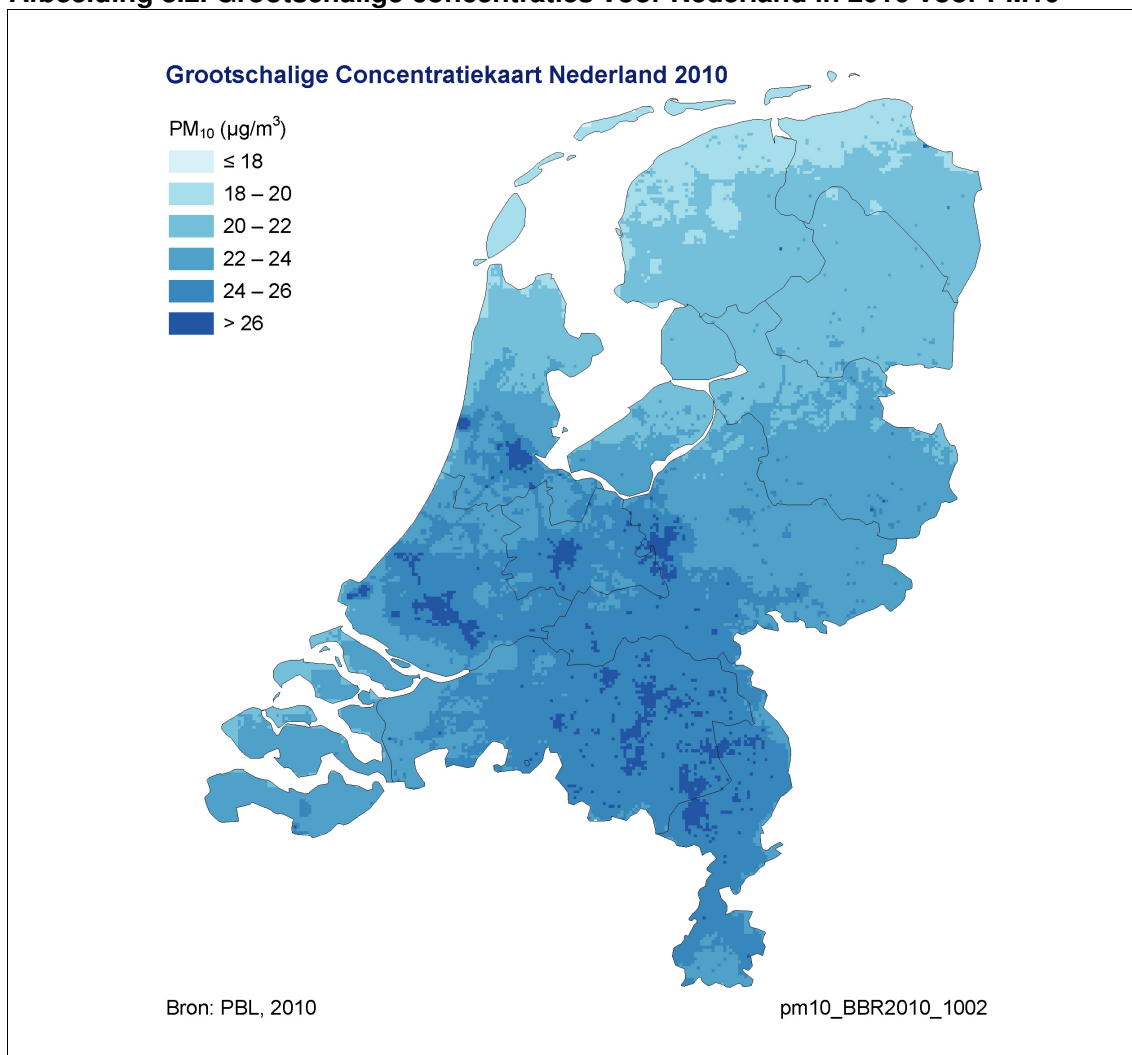
Afbeelding 8.2. Grootschalige concentraties voor Nederland in 2010 voor PM 10
