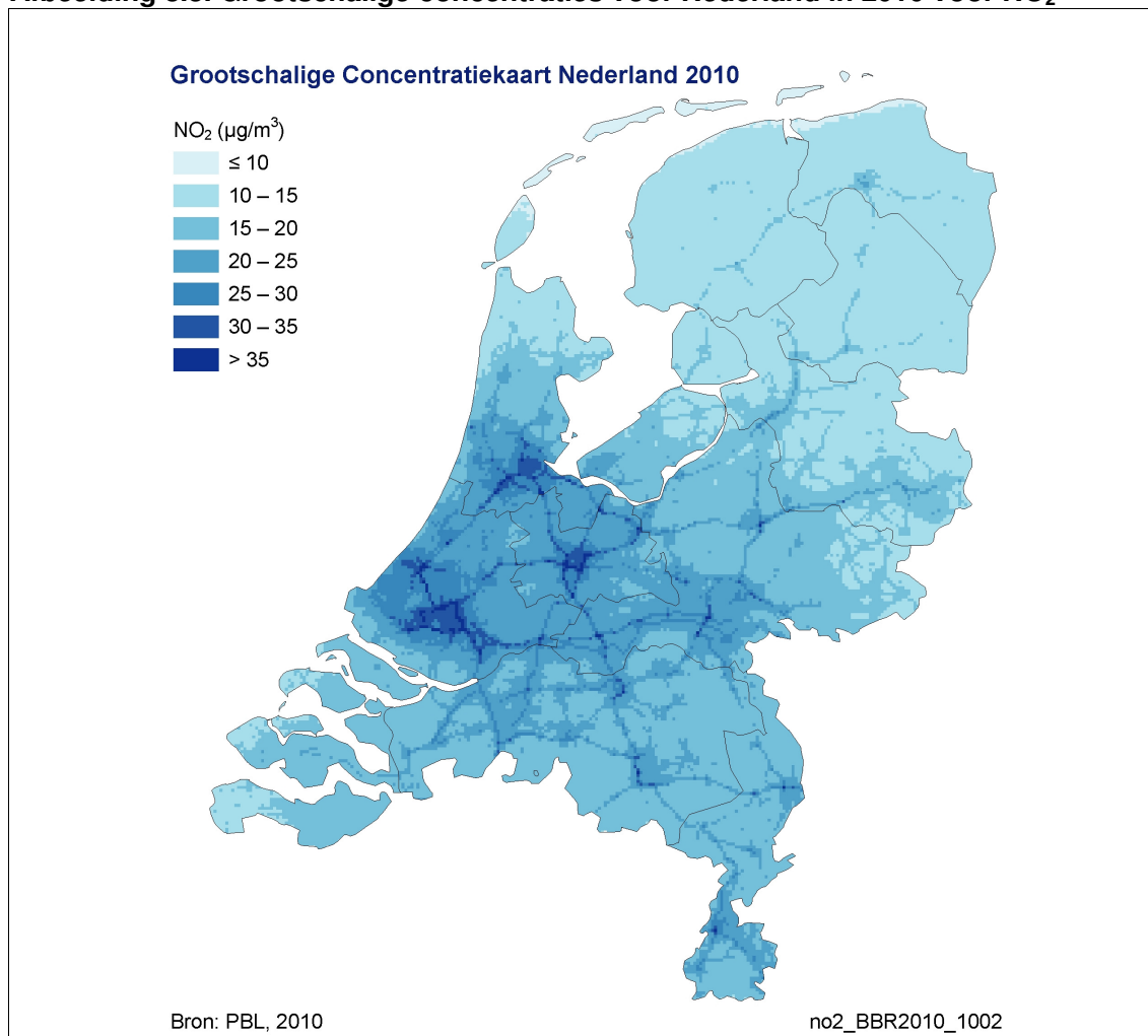
Afbeelding 8.3. Grootschalige concentraties voor Nederland in 2010 voor NO 2
