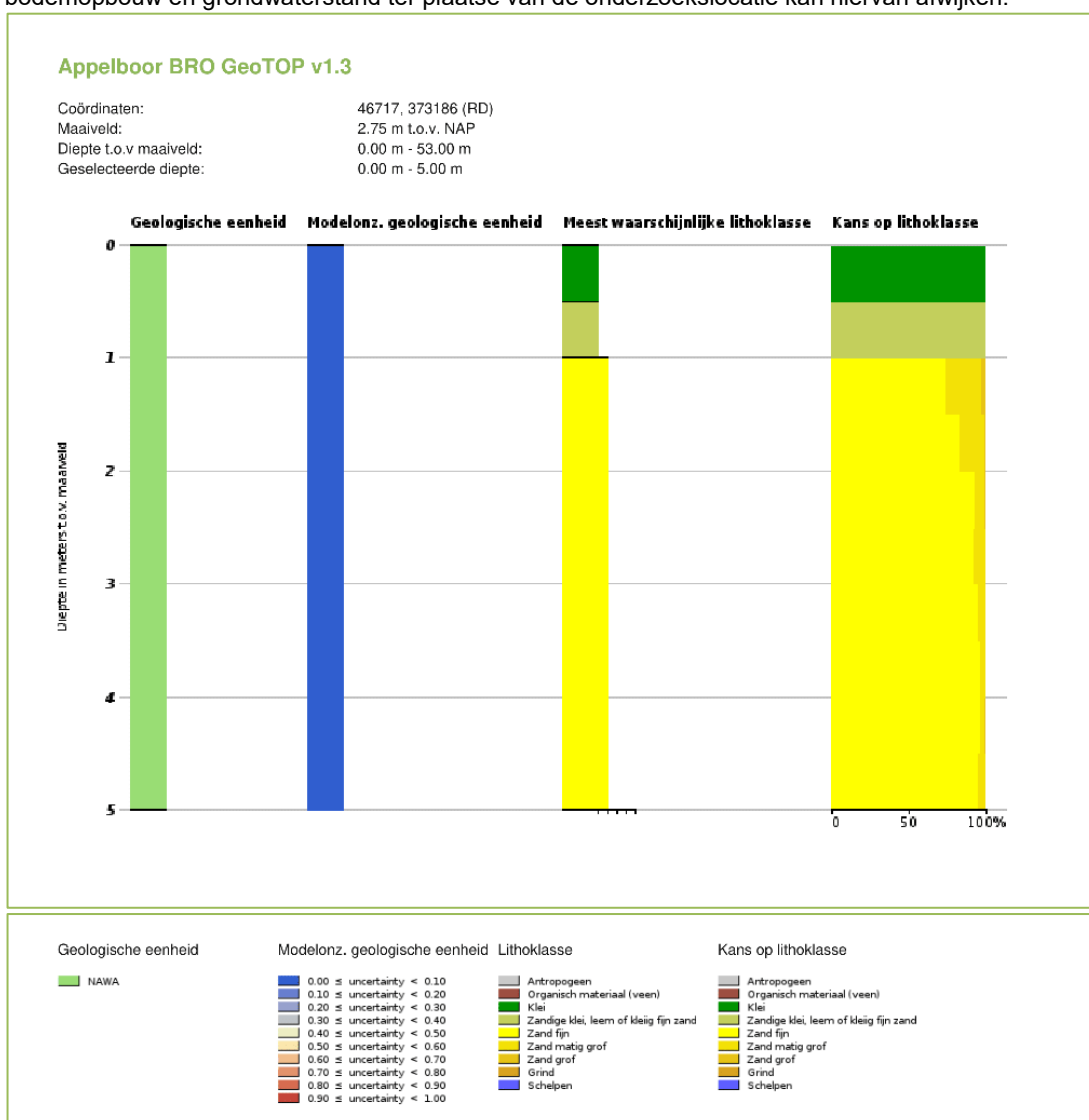
Figuur 2.1 Gemodelleerde bodemopbouw tot 5 m-mv.
