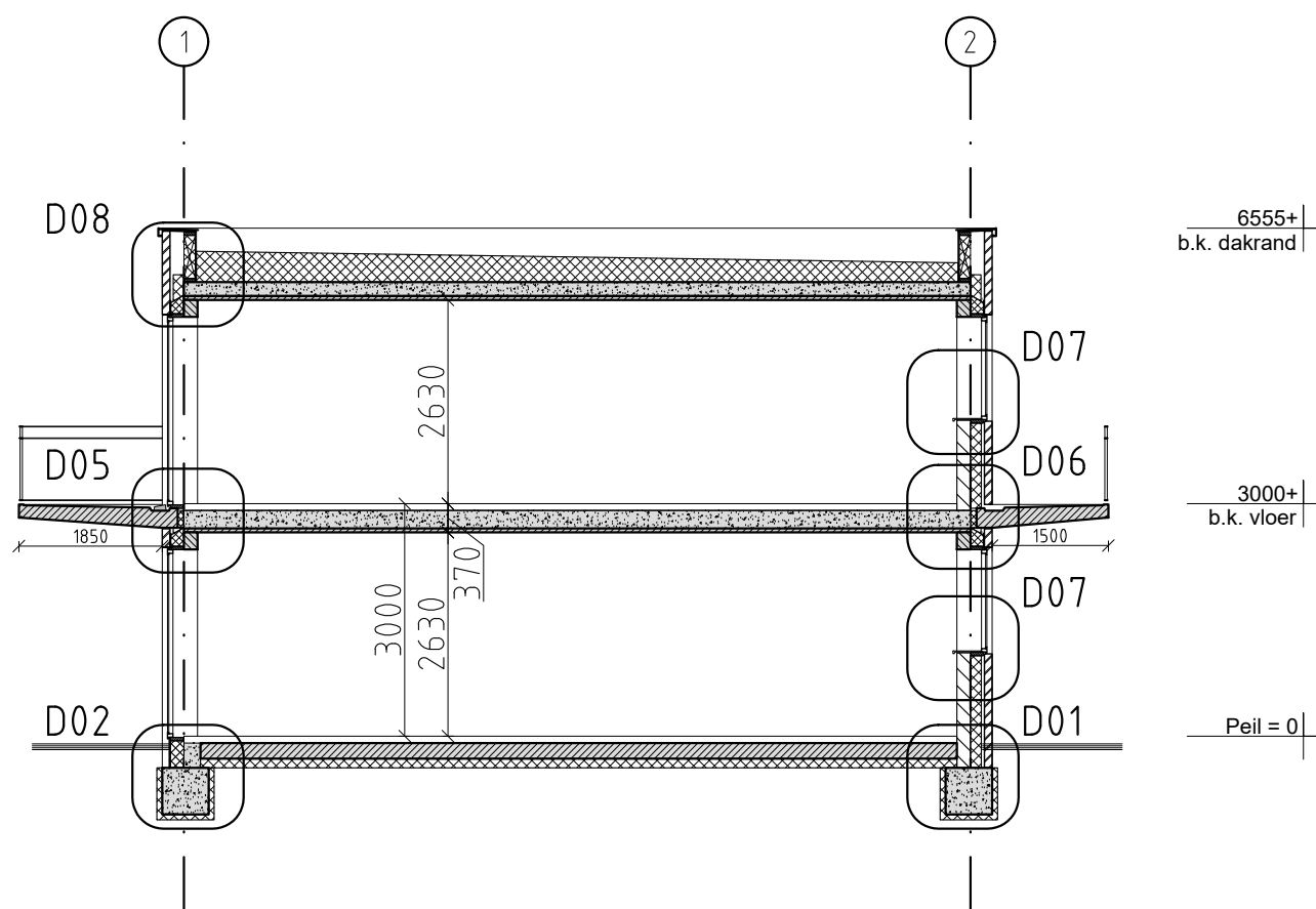
DOORSNEDE A-A
