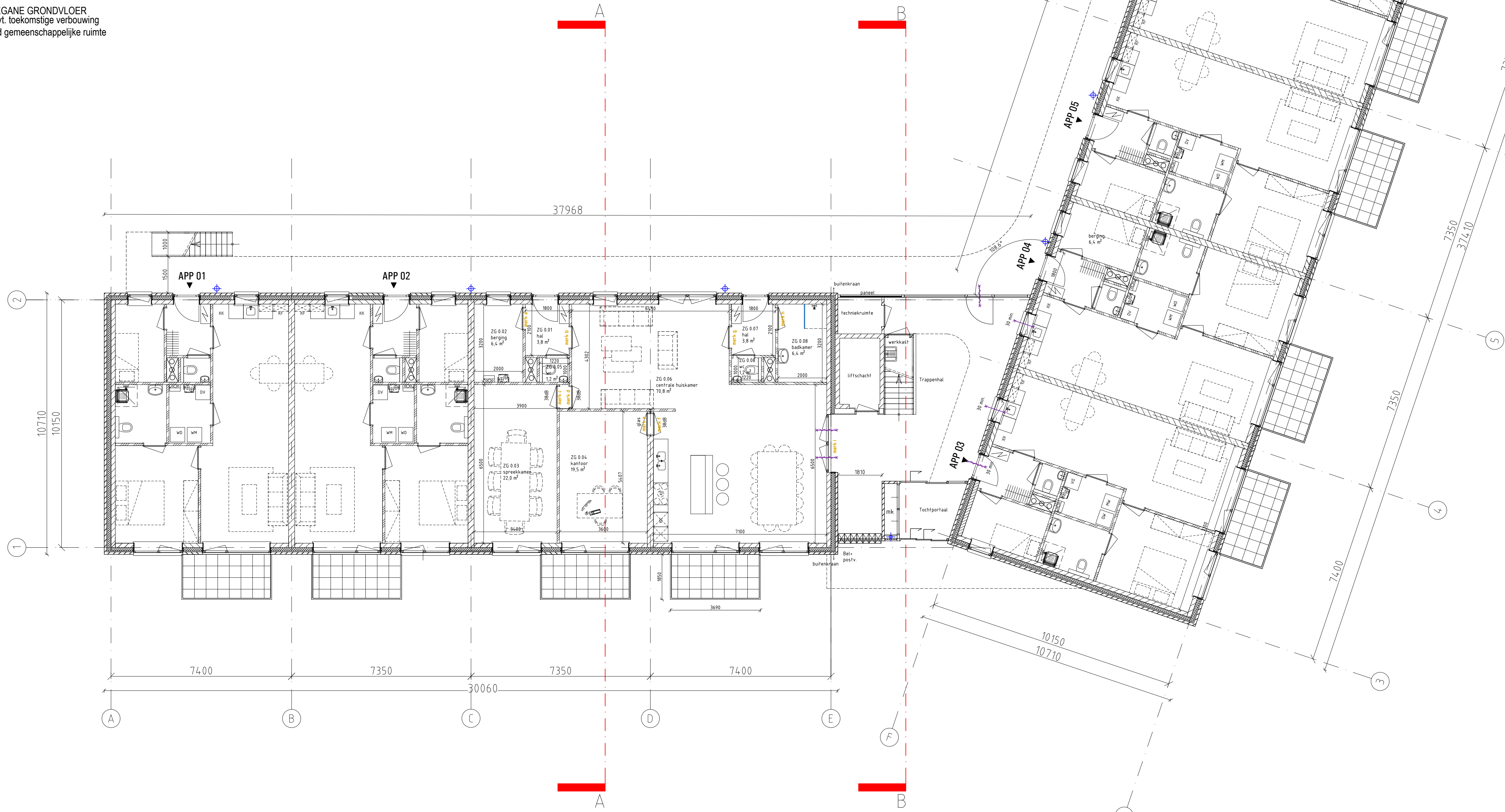
BEGANE GRONDVLOER
