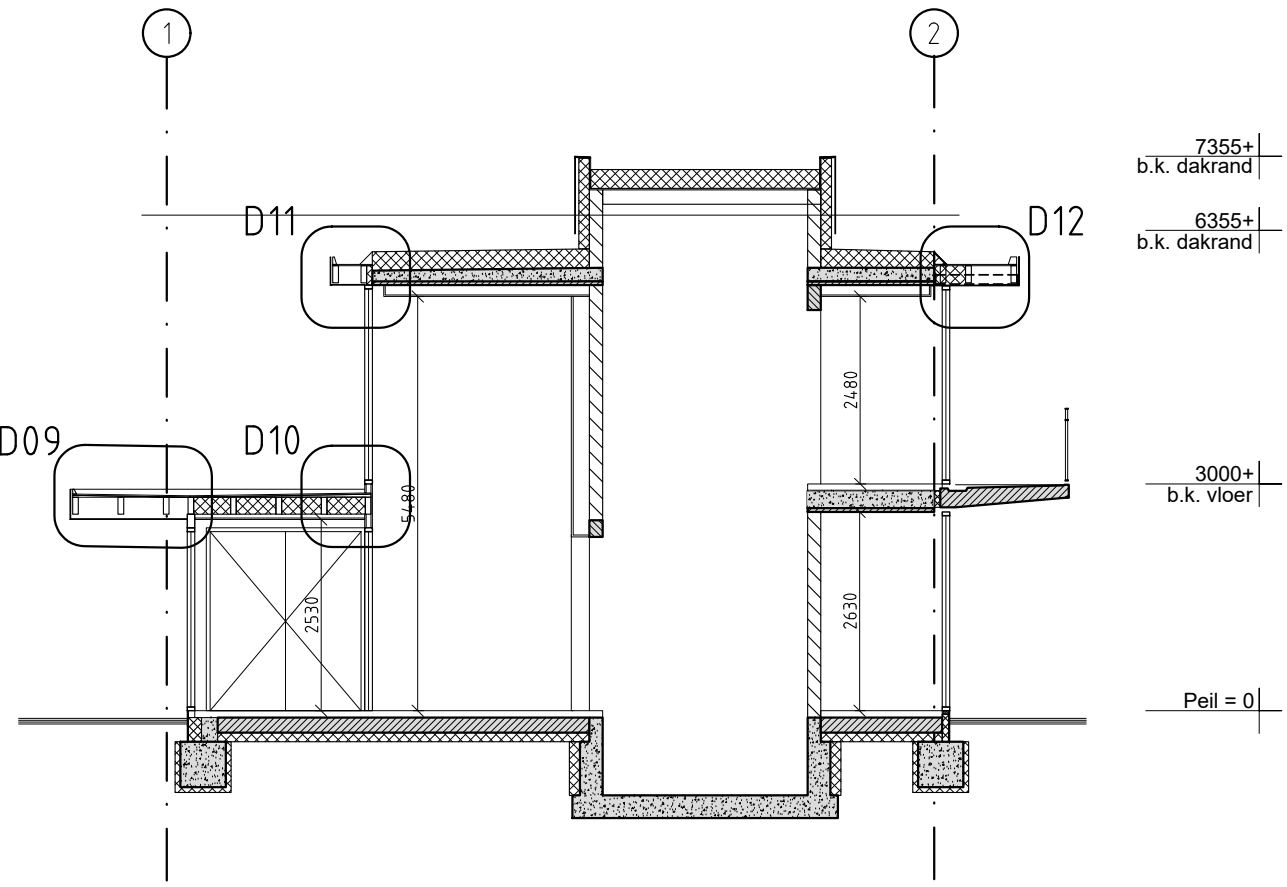
DOORSNEDE B-B
