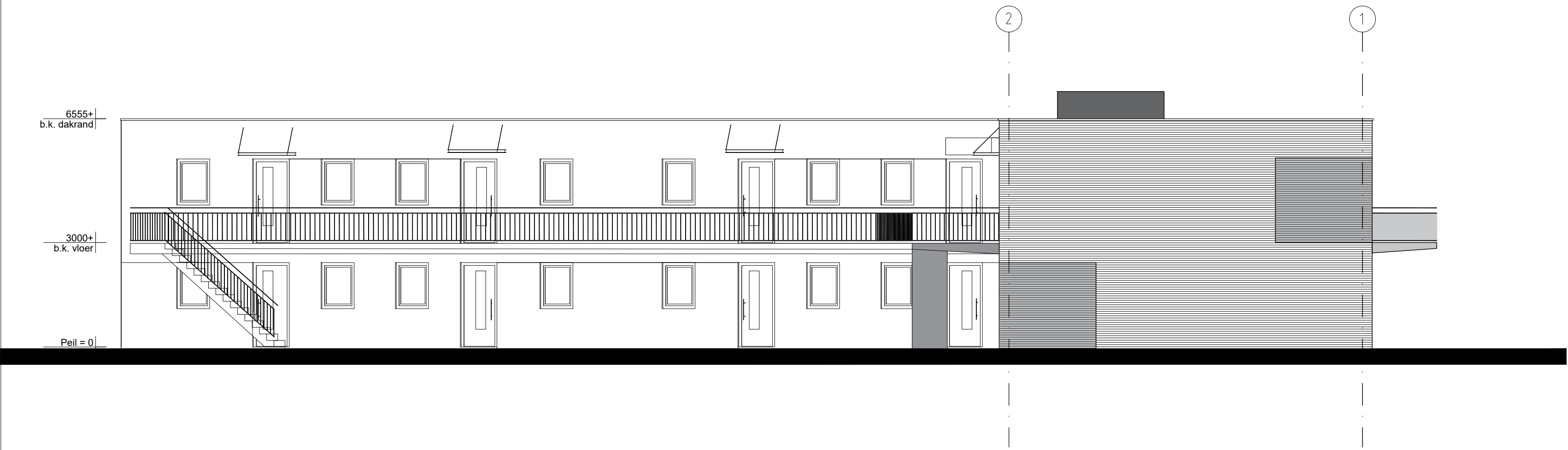
LINKER ZIJGEVEL BLOK A 06
