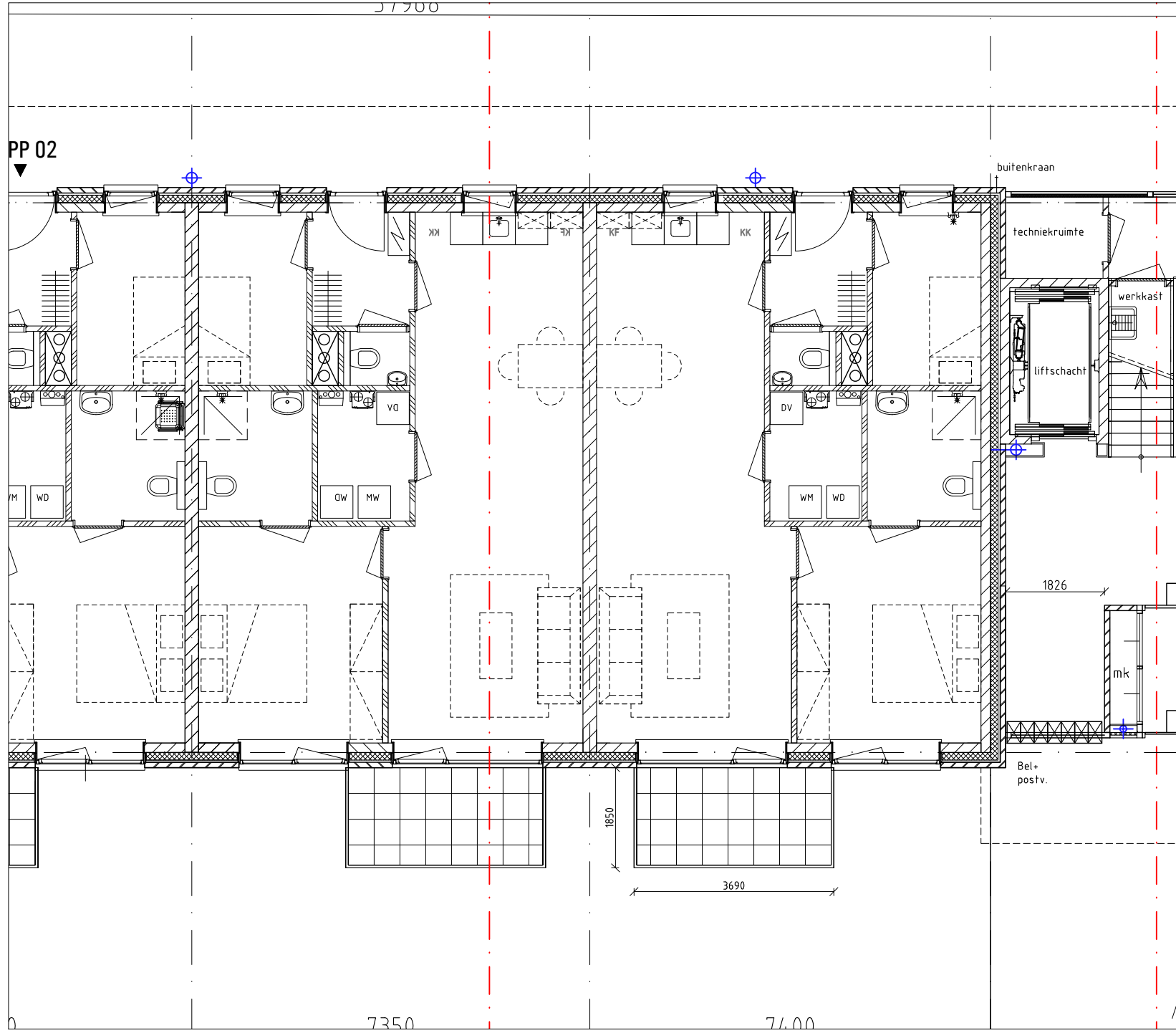
BEGANE GRONDVLOER evt. toekomstige verbouwing vd gemeenschappelijke ruimte
