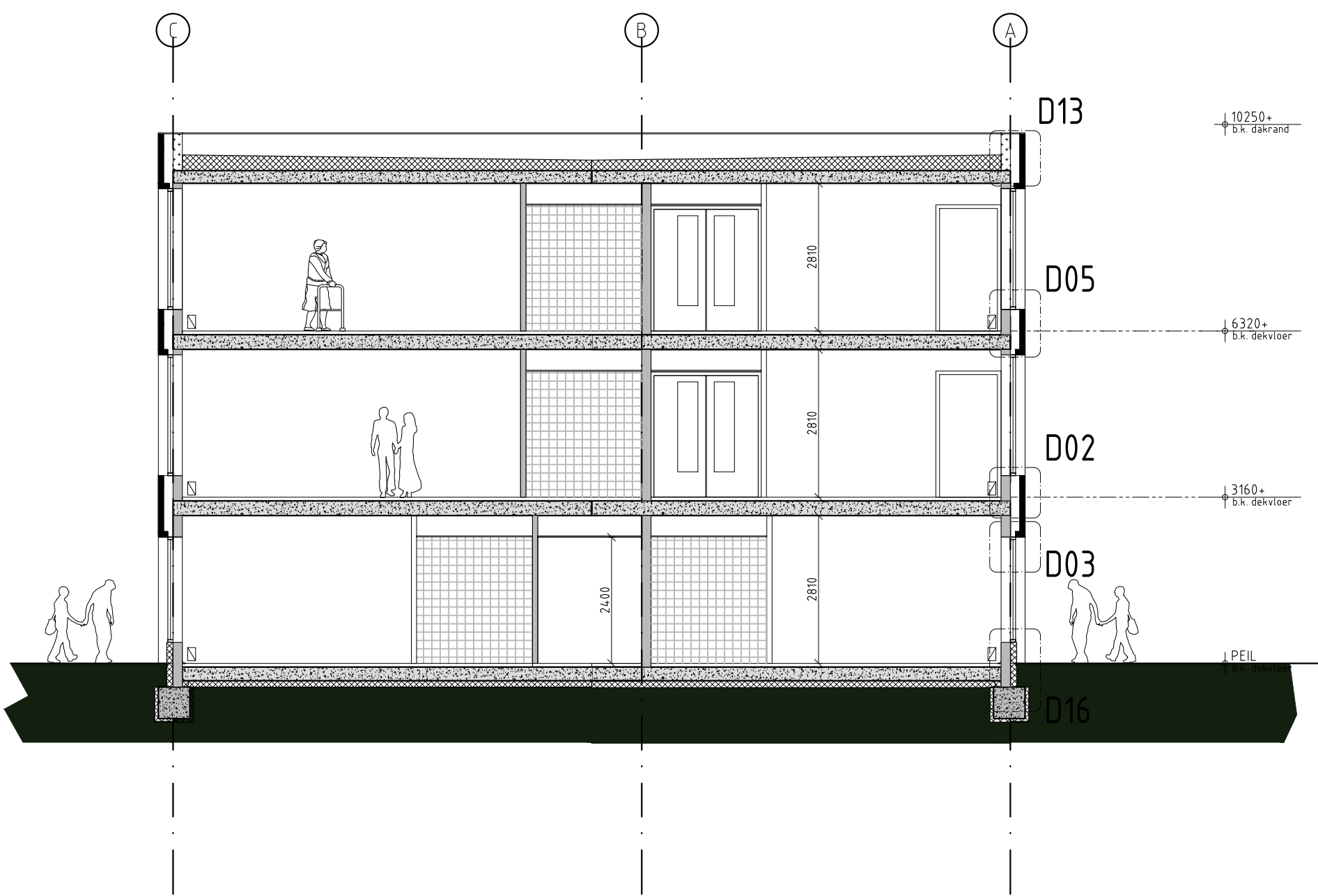
DOORSNEDE BB 1:100
