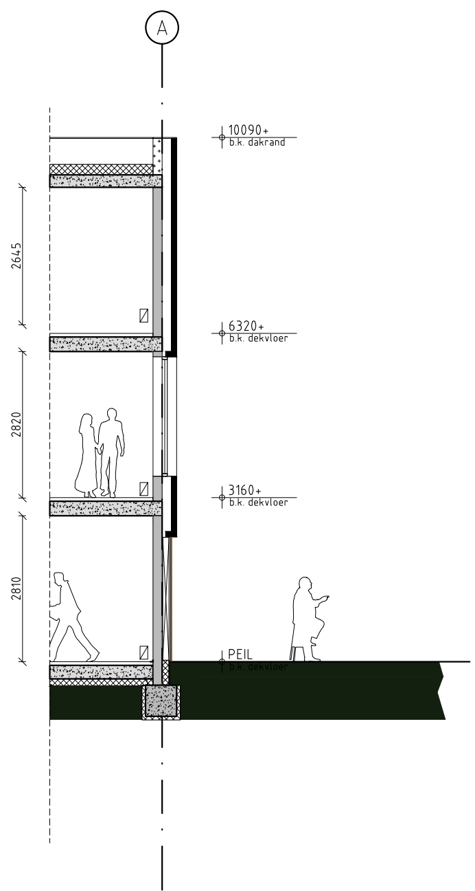
DOORSNEDE D 1:100
