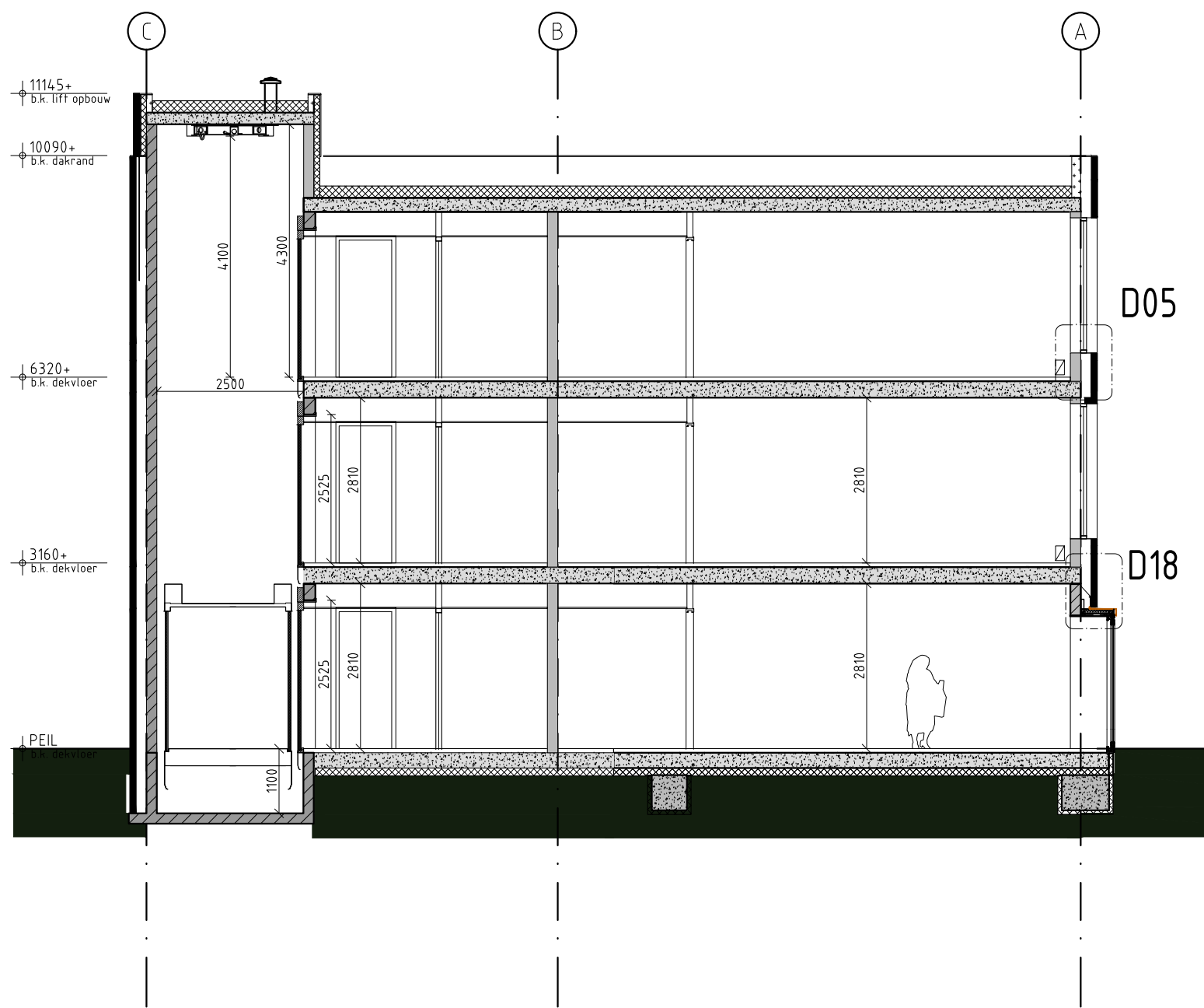
DOORSNEDE FF 1:100
