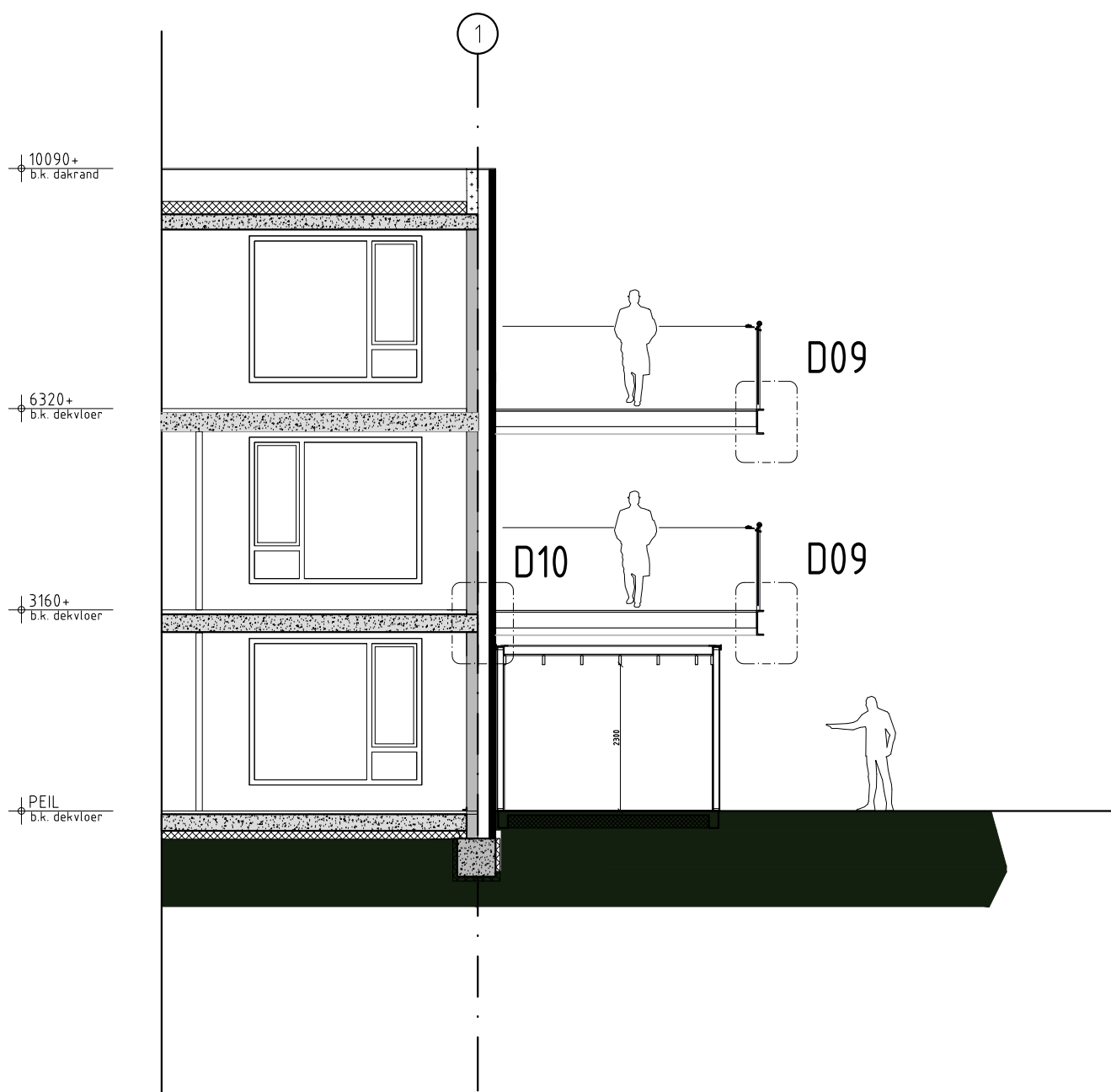
DOORSNEDE E 1:100
