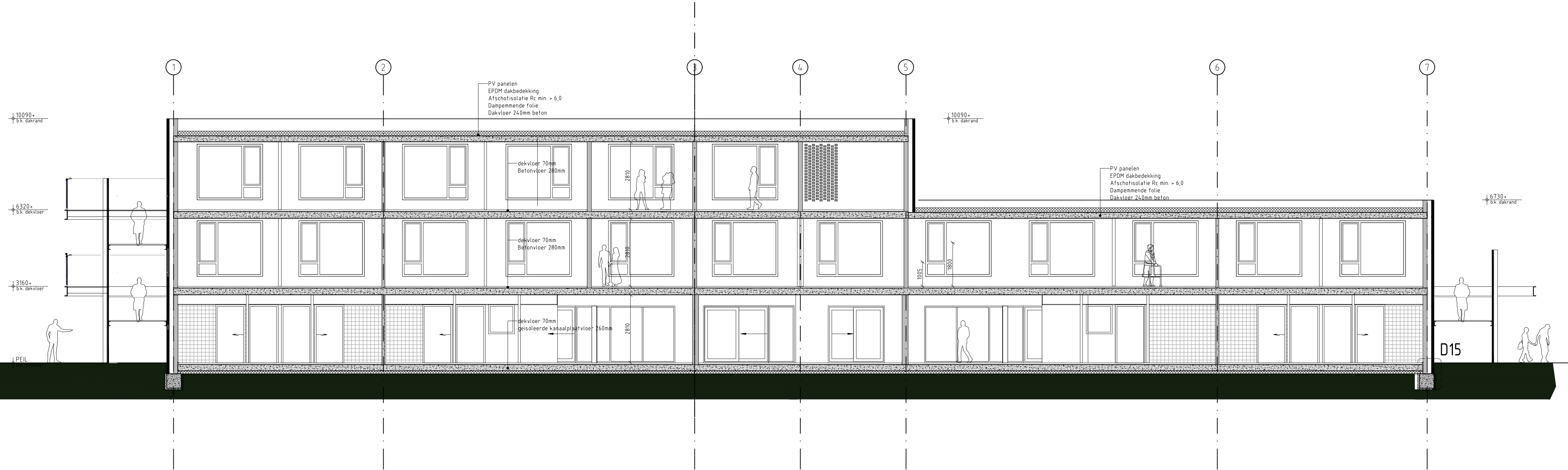
DOORSNEDE AA 1:100
