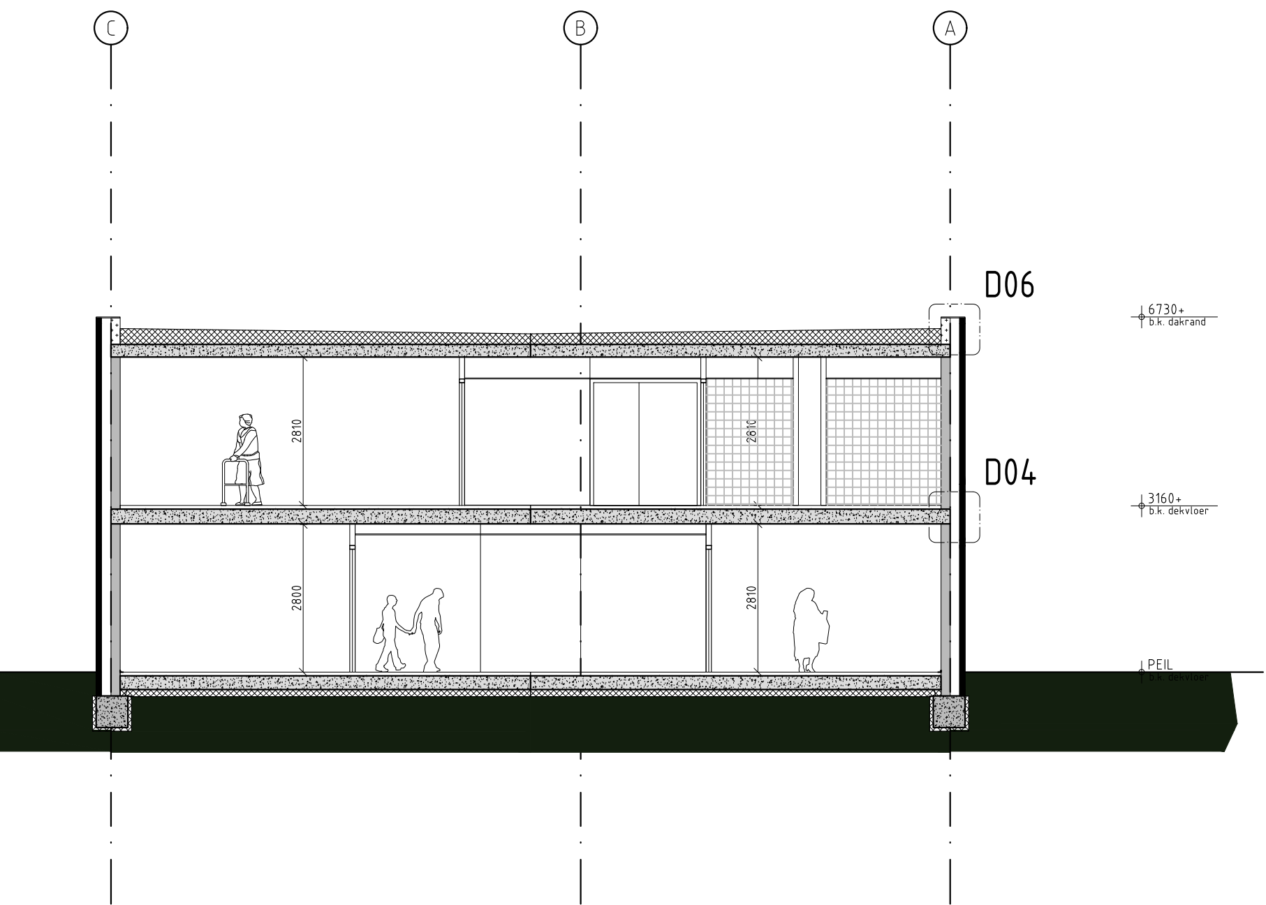
DOORSNEDE CC 1:100
