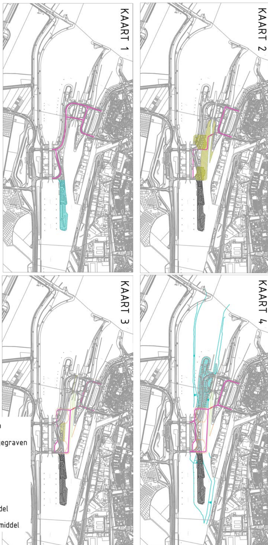
Figuur 5-7 Uitvoeringsplanning variant 1
