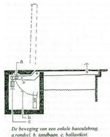
Figuur 5-3 Basculebrug met 1 val
