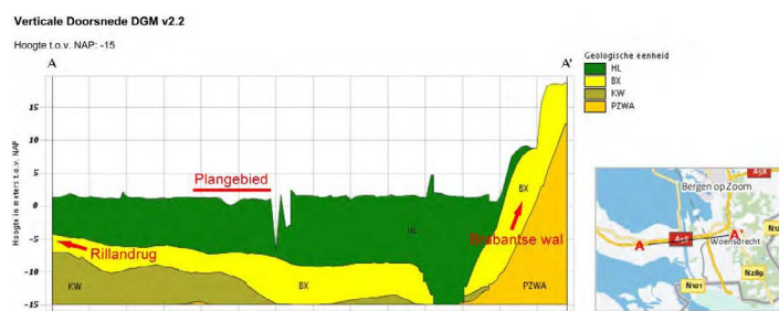
Afbeelding 9 Afbeelding 13 Geologisch model tot 15 meter –NAP op basis van DGM v2.2 tussen Reimers-waal en Woensdrecht. Bron: Geologische Dienst Nederland – TNO, 2014
