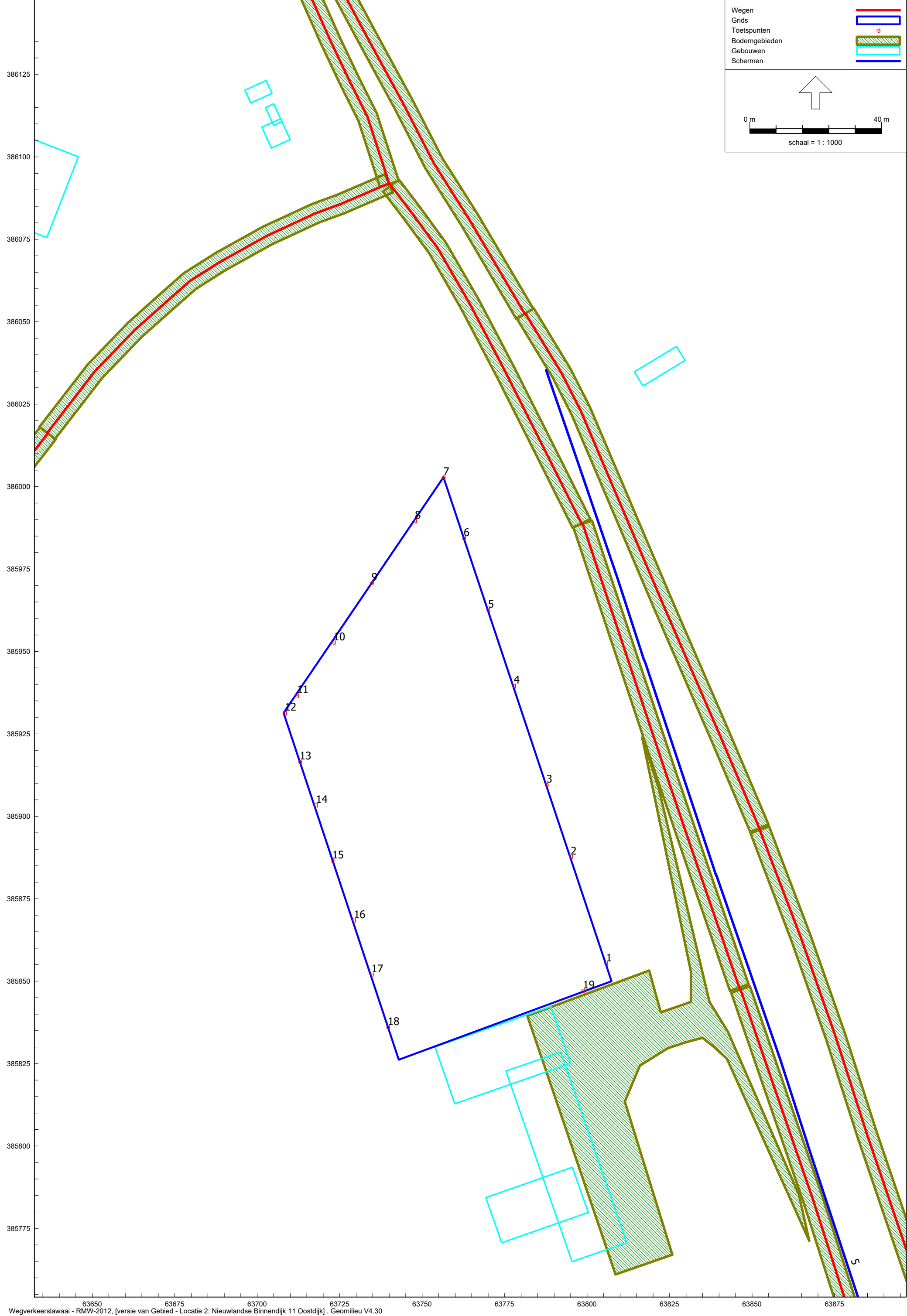
Figuur 2B: grafisch overzicht rekenpunten locatie 2 Vlax Akoestiek en Lawaai beheersing
