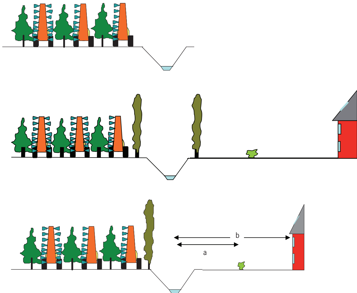
Figuur 6. Drie situaties; met sloot, met/zonder windhaag, met standaard of driftarme boomgaard spuit, met 3 m of 9 m teeltvrije zone met aangegeven de afstanden van perceelsgrens tot a. rand achtertuin (0-3 m hoogte blootstelling) en b. gevel bebouwing (3-6 m blootstelling).
