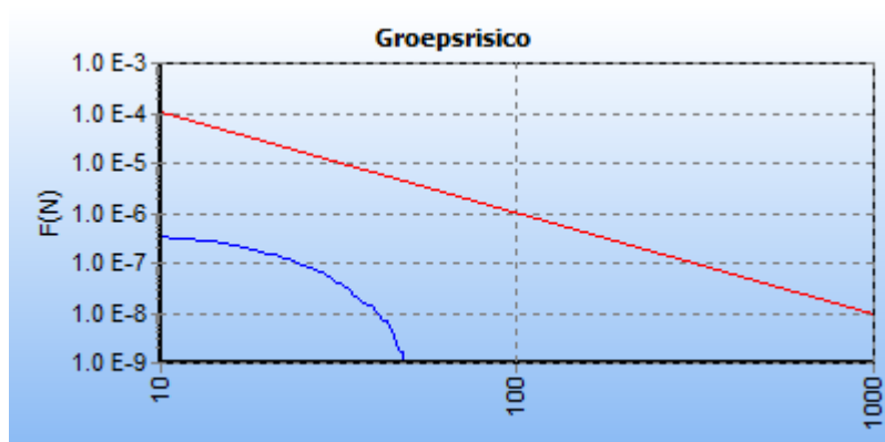
Figuur 5.6 FN-Curve W-528-01 huidige situatie
