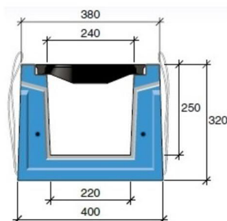
Figuur 11 Afmetingen HRI 300 roostergoot
