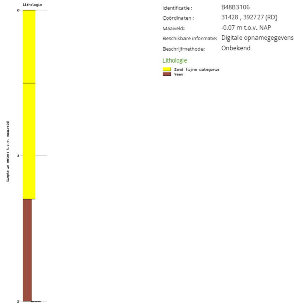
Boormonsterprofiel
