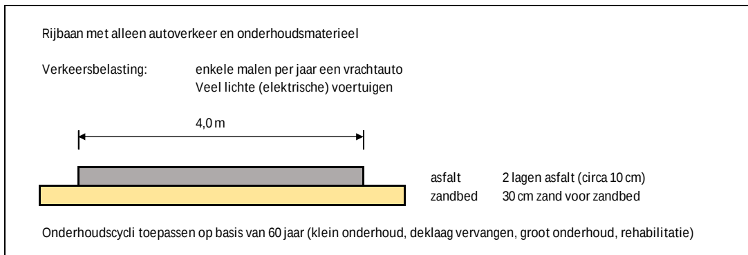
Figuur 3-2 0+ variant profiel 'rijbaan met autoverkeer en onderhoudsmaterieel'
