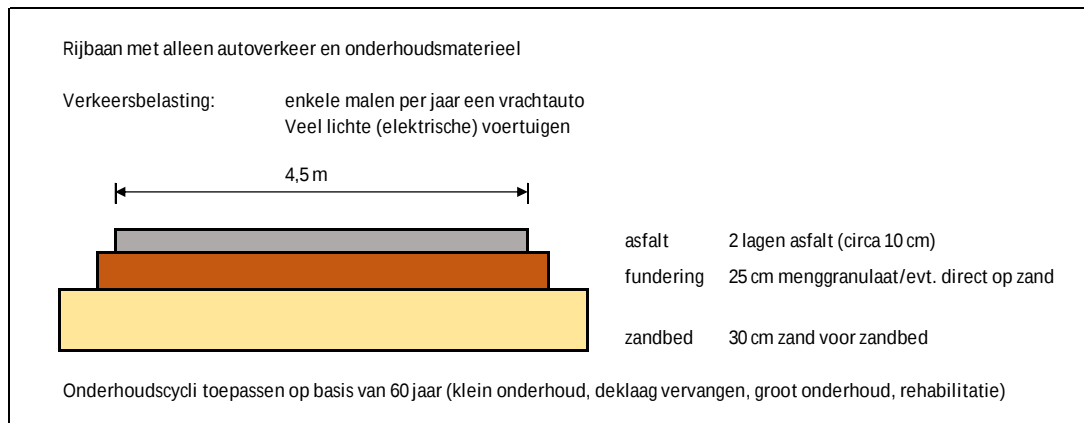
Figuur 2-2 Grafische weergave profiel 'Rijbaan met alleen autoverkeer en onderhoudsmaterieel'
