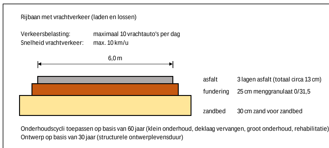
Figuur 2-1 Grafische weergave profiel 'Rijbaan met vrachtverkeer'
