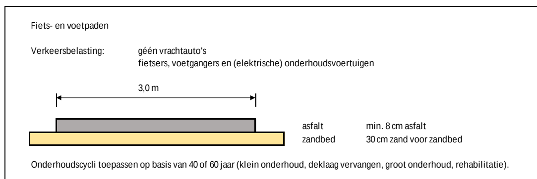
Figuur 3-4 0+ variant profiel 'fiets- en voetpaden'
