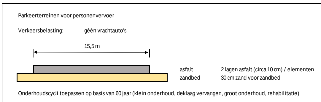
Figuur 3-3 0+ variant profiel 'parkeerterreinen voor personenvervoer'
