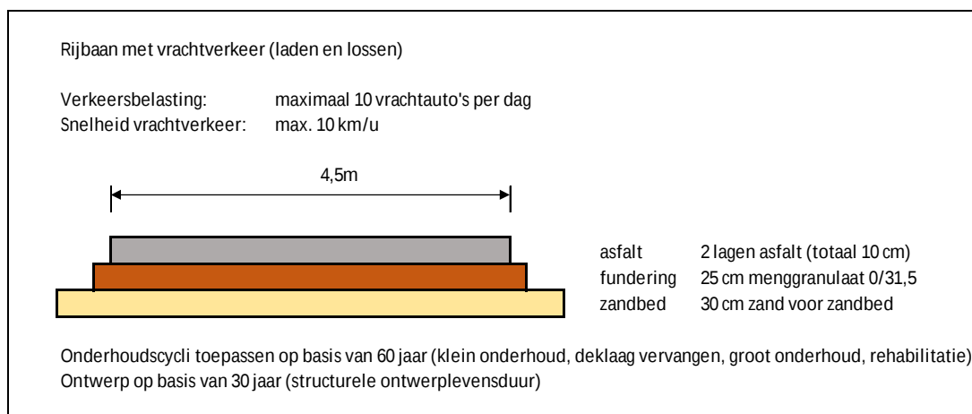
Figuur 3-1 0+ variant profiel 'Rijbaan met vrachtverkeer'
