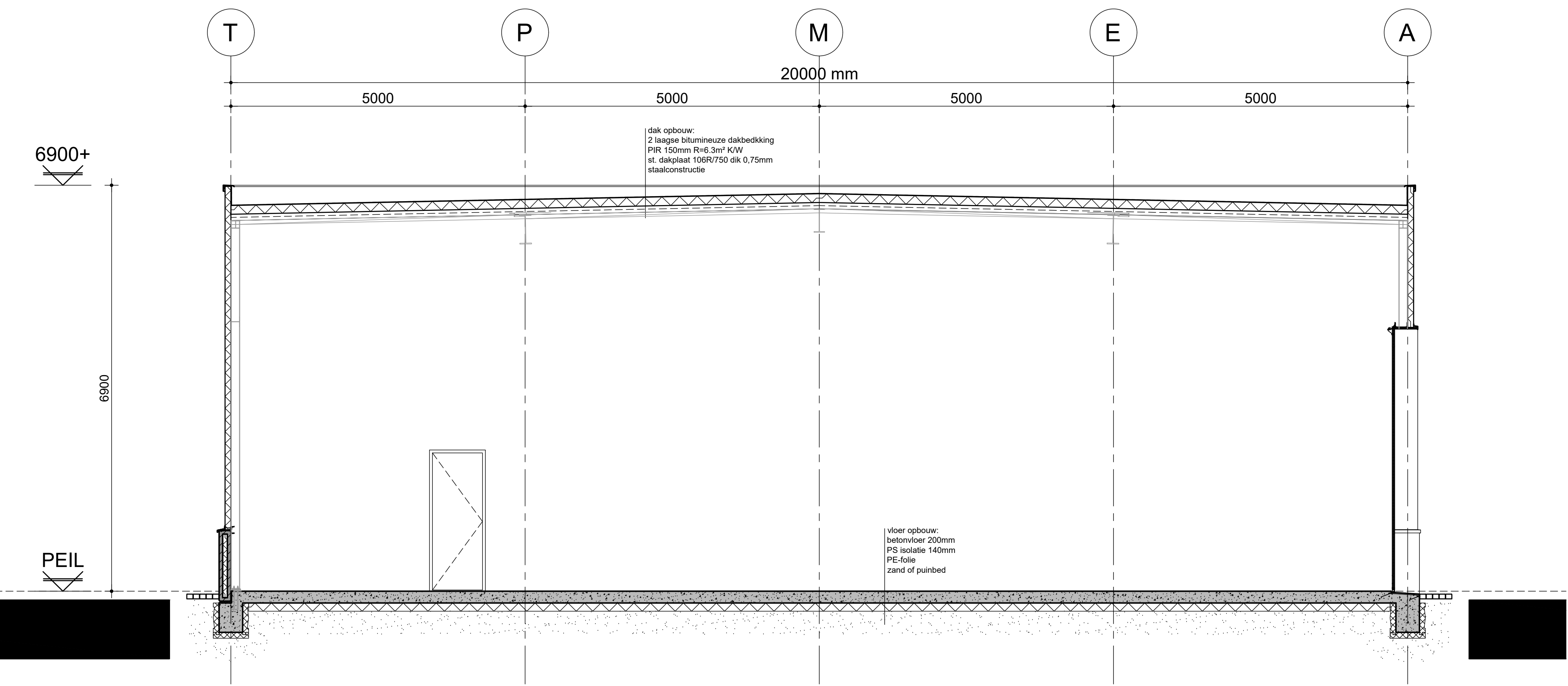
doorsnede A-A
