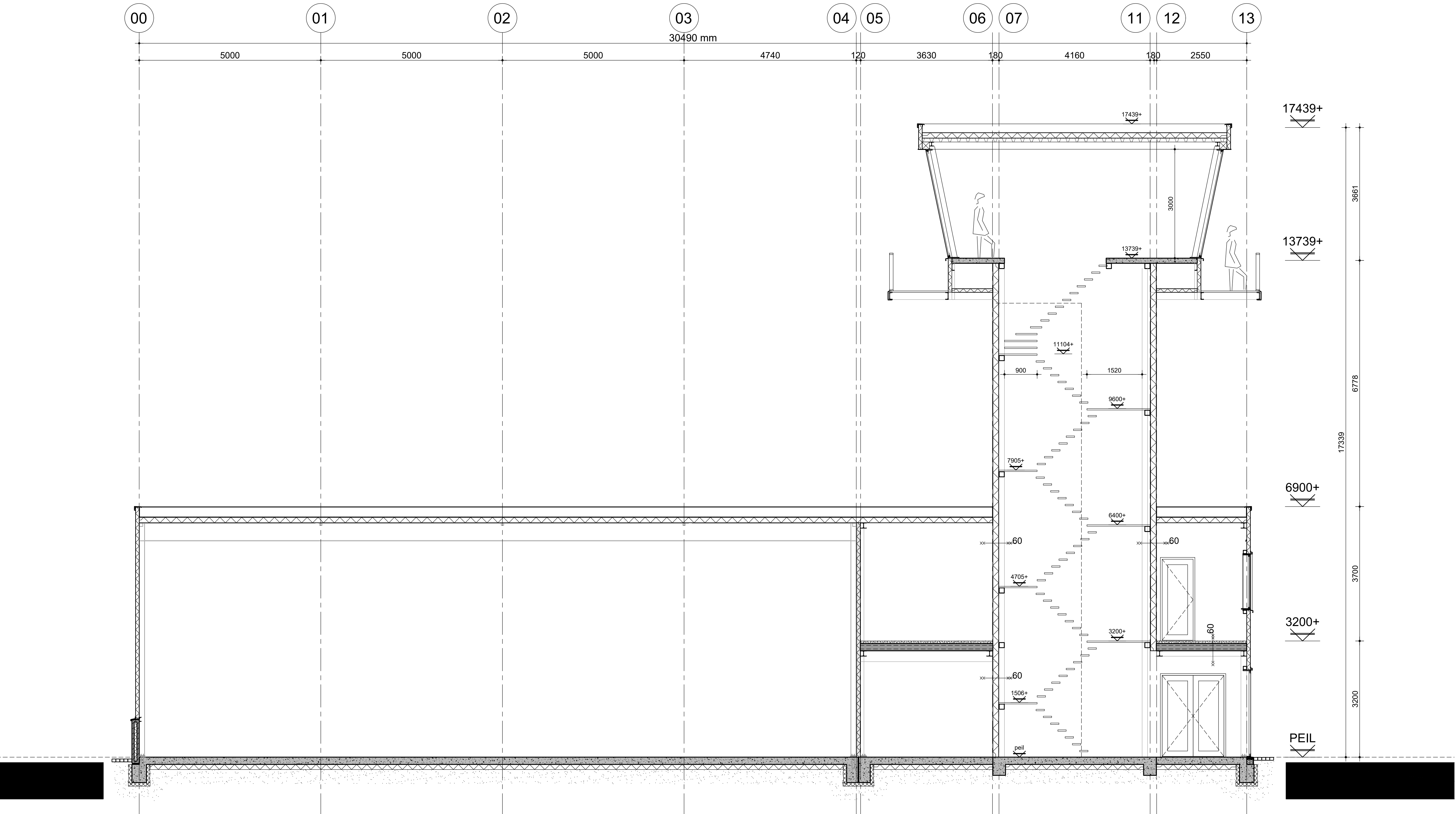
doorsnede B-B
