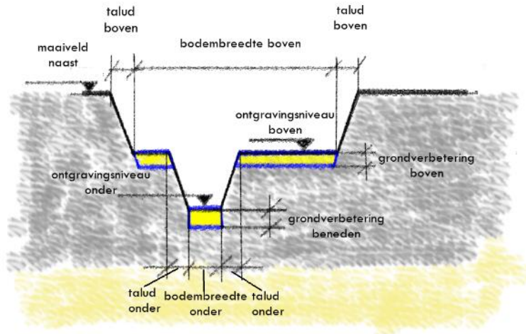
figuur 8 – schets doorsnede ontgraving met begrippen
