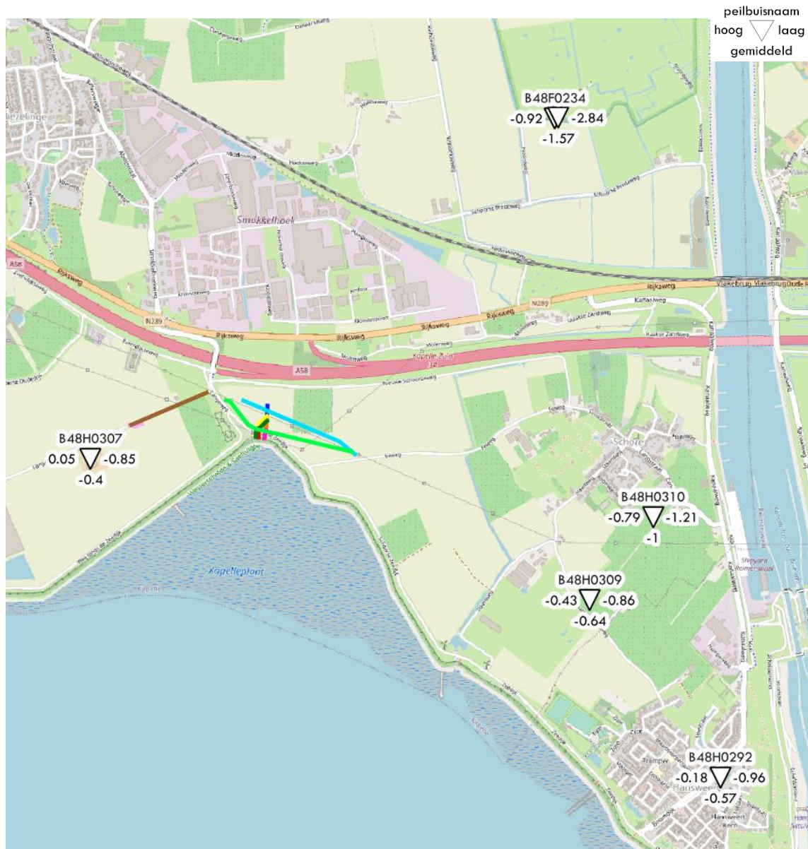
figuur 7 - grondwaterstand t.o.v. NAP per geanalyseerde peilbuis (wit = freatisch/watervoerende laag 1, rood = watervoerende laag 3)
