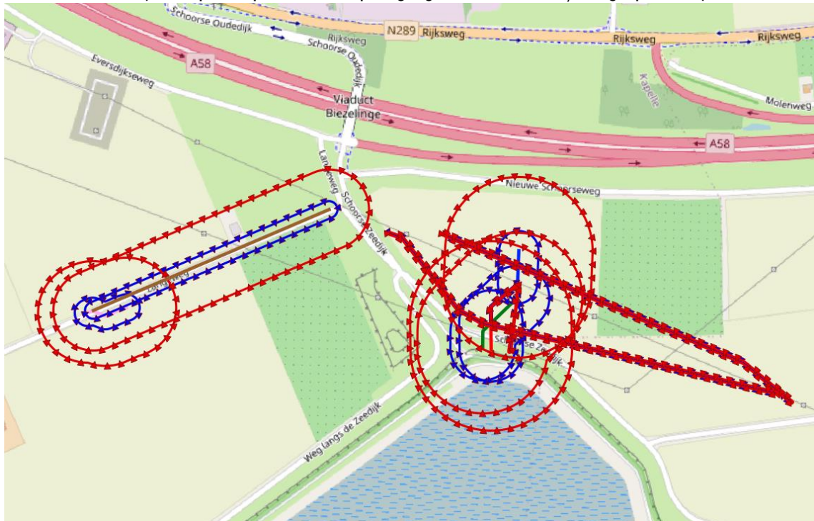
figuur 5 – reikwijdte bemaling, grootste reikwijdte per watervoerende laag is gebruikt voor deze figuur (blauw=prognose onder normale omstandigheden, rood=extreem bij een natuurlijk lage grondwaterstand/droge periode)
