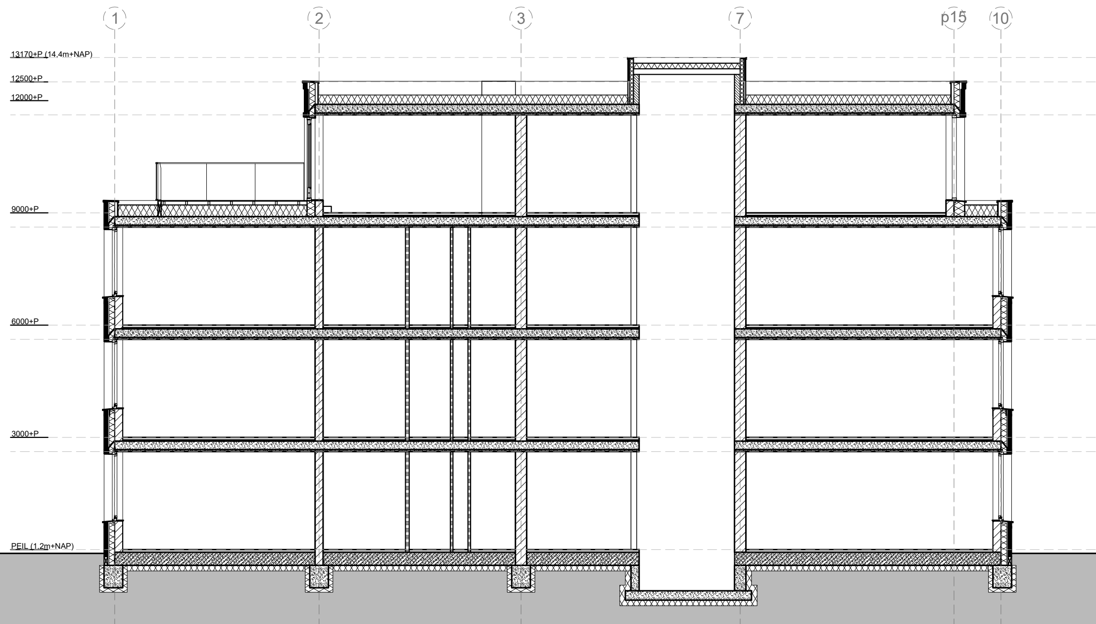
principe doorsnede appartementen
