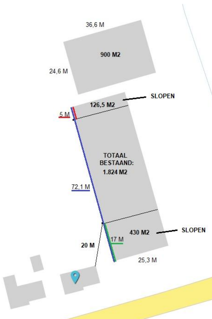
Gemaatvoerde tekening bestaande situatie
