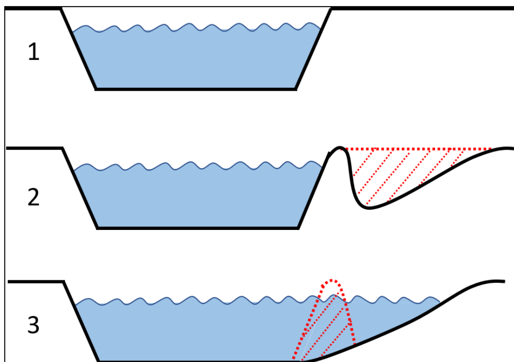
Figuur 6 Schematische weergave van de werkwijze voor het uitgraven van nieuwe watergangen.
