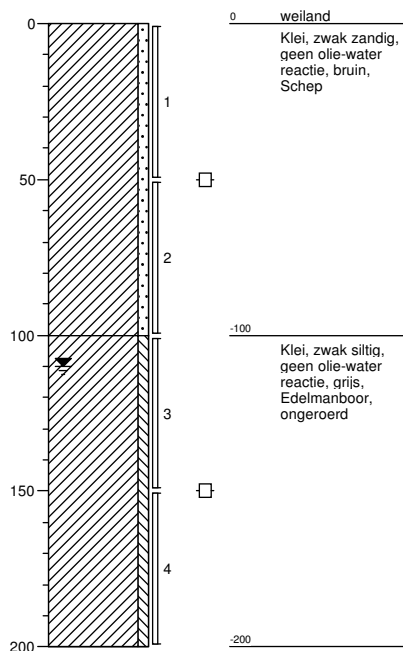
Boring: 04 boormeester Jtiben Sleuflengte [m]: 0,3 Sleufbreedte [m]: 0,3
