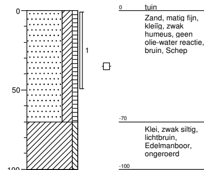
Boring: 03 boormeester Jtiben Sleuflengte [m]: 0,3 Sleufbreedte [m]: 0,3
