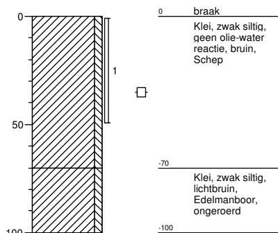
Boring: 05 boormeester Jtiben Sleuflengte [m]: 0,3 Sleufbreedte [m]: 0,3
