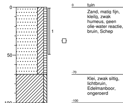
Boring: 06 boormeester Jtiben Sleuflengte [m]: 0,3 Sleufbreedte [m]: 0,3
