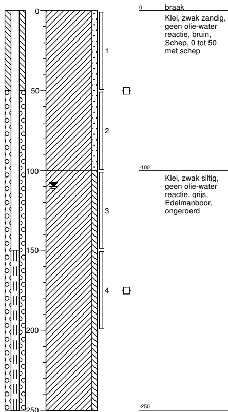
Boring: 01 boormeester Jtiben Sleuflengte [m]: 0,3 Sleufbreedte [m]: 0,3
