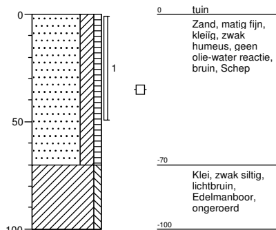
Boring: 02 boormeester Jtiben Sleuflengte [m]: 0,3 Sleufbreedte [m]: 0,3
