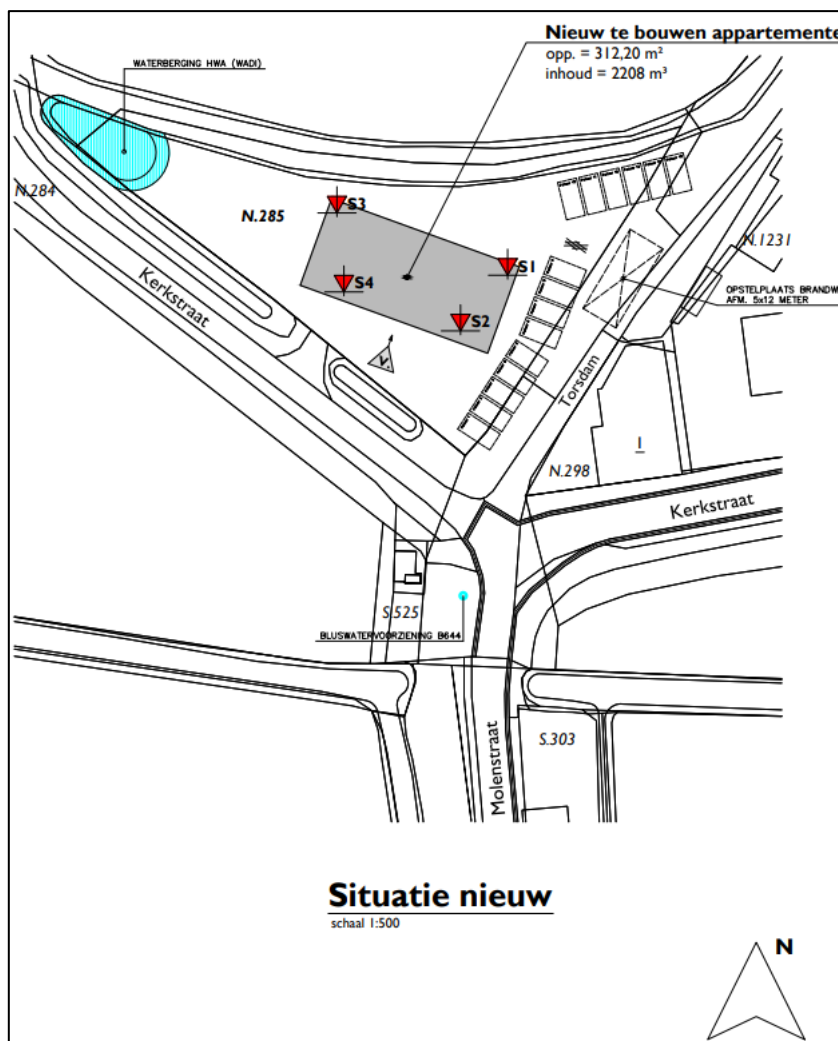
Figuur 1.4 Visuele representatie van de beoogde situatie (bron: Bouwbureau van Rossum).
