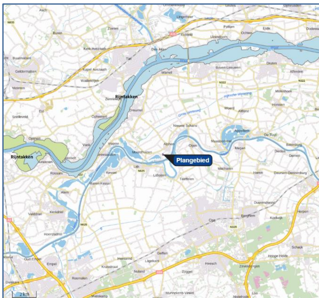
Afbeelding 2. Ligging van het plangebied ten opzichte van Natura 2000-gebieden
