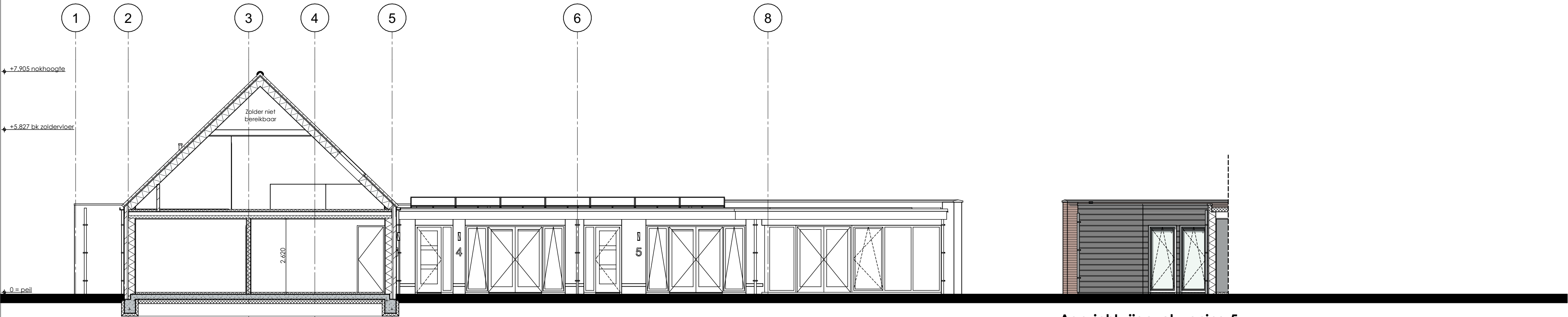
Doorsnede B-B
