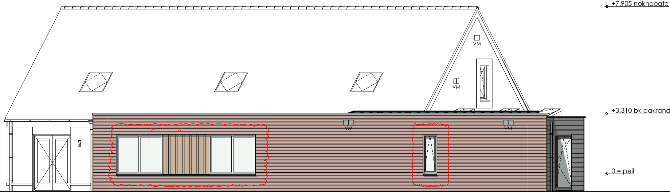
Rechtergevel (noord-oost)
