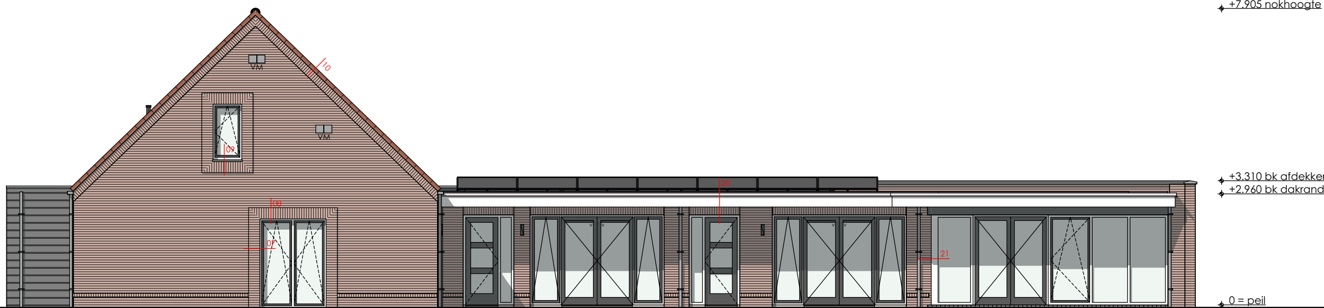
Voorgevel (zuid-west)
