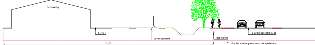
Dwarsprofiel gasleiding 1:200
