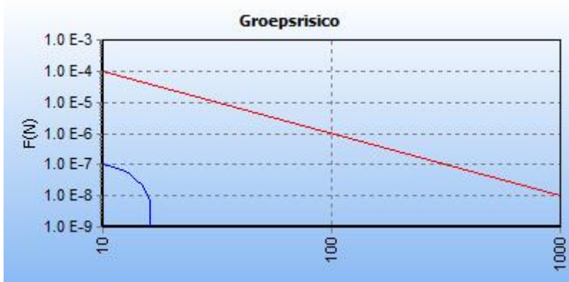
5.2 Figuur 5.2 FN curve voor 6657_leiding-Z-567-23-deel-1 van N.V. Nederlandse Gasunie voor de kilometer tussen stationing 1740.00 en stationing 2740.00
