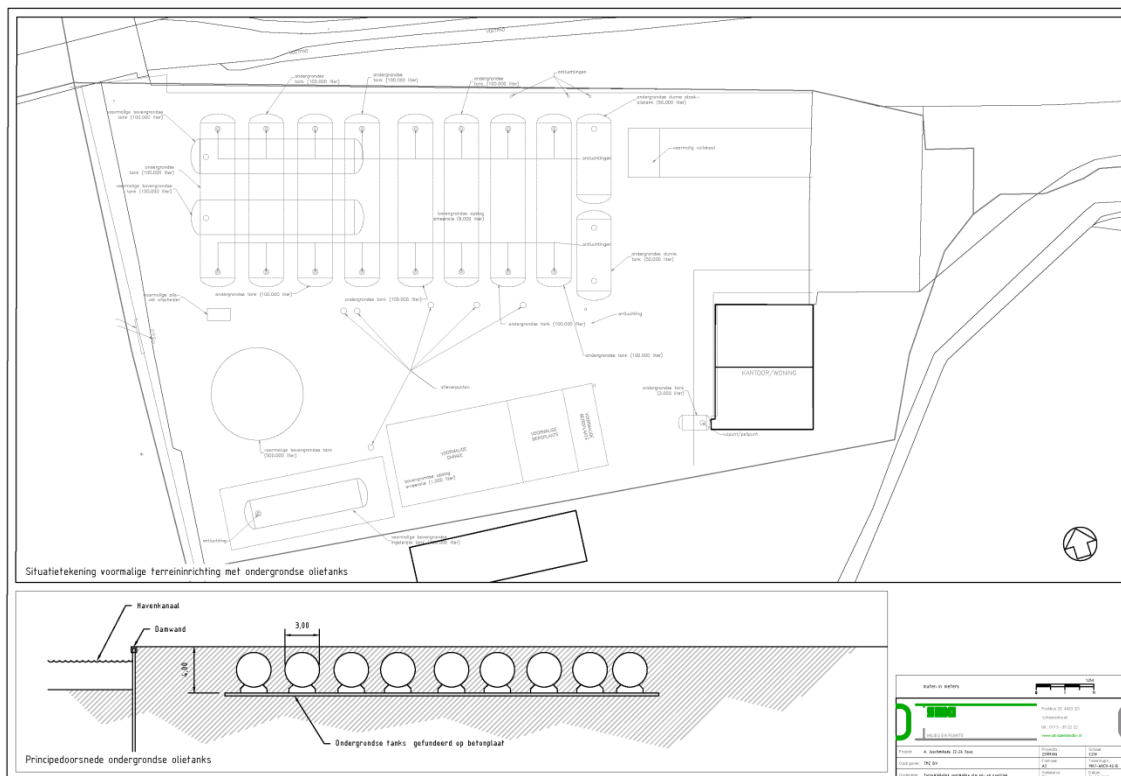
Situatietekening oorspronkelijke terreininrichting oliehandel Van der Dries met principedoorznede van de nog in de bodem aanwezige ondergrondse olietanks
