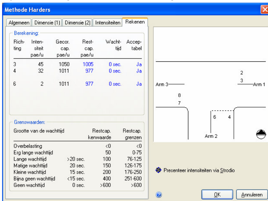
Afbeelding 9 Capaciteitsberekening Oud Ovezandseweg – Mr. Dr. Messtraat
