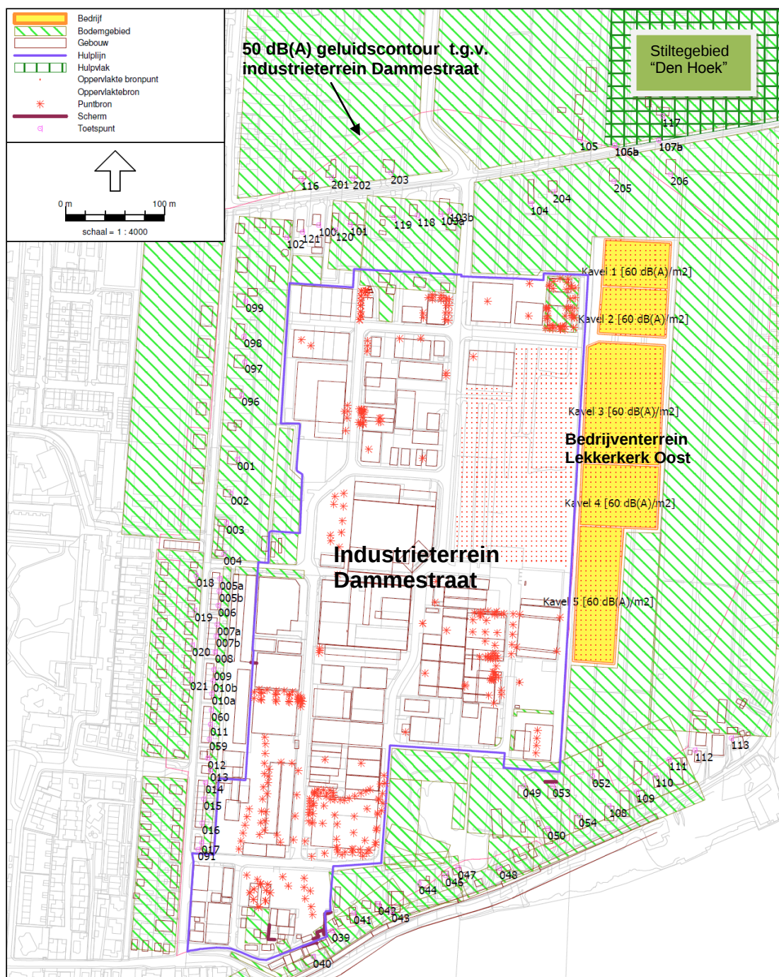
Figuur 3: Overzicht rekenmodel met indeling kavels en de kentallen per kavel (de figuur is niet op schaal).
