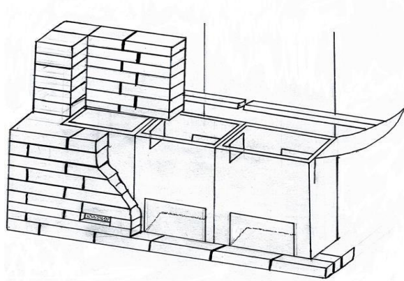
Doorsnede Ingemetselde vleermuisvoorzieningen Buitenaanzicht in pandige voorzieningen.
