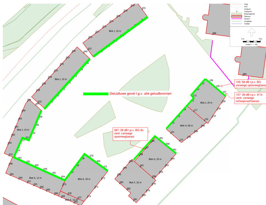
Figuur 3: Overzicht geluidluwe gevels.
