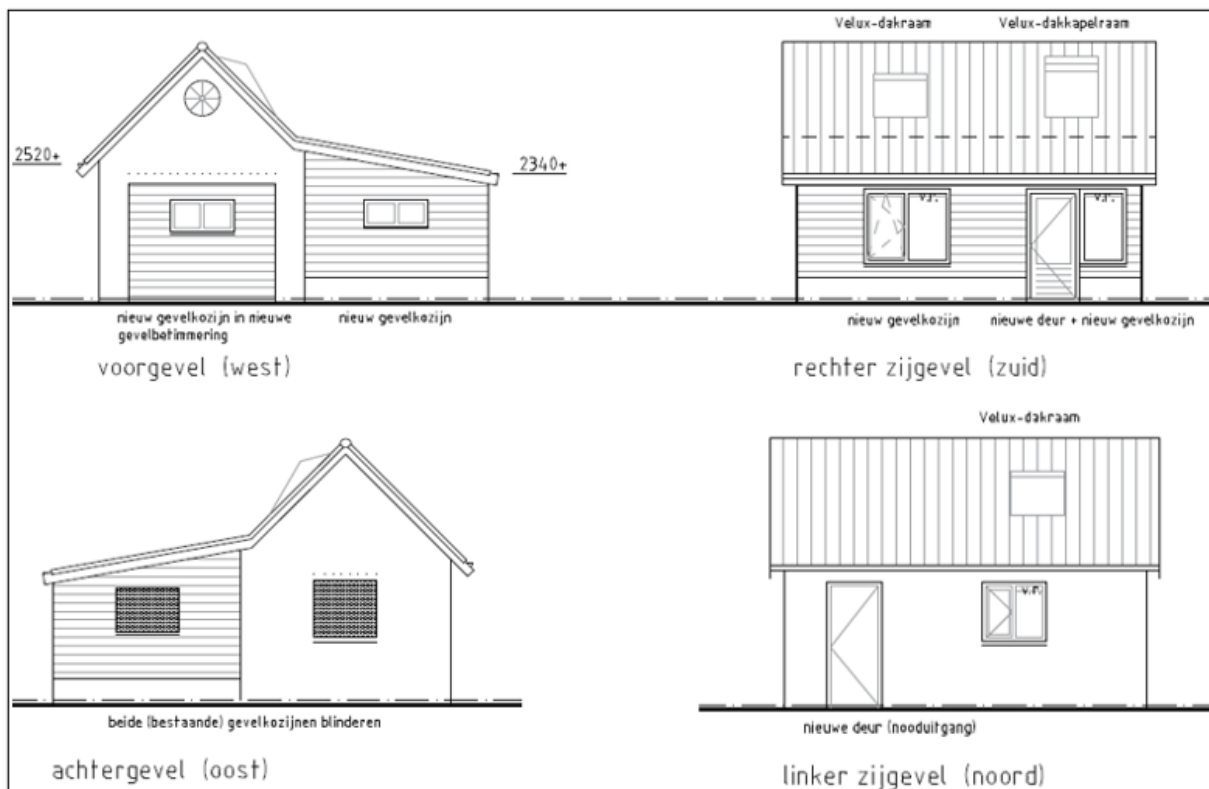
Aanzichttekeningen nieuw.
