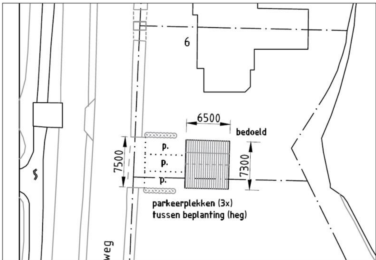
Situatietekening nieuw.
